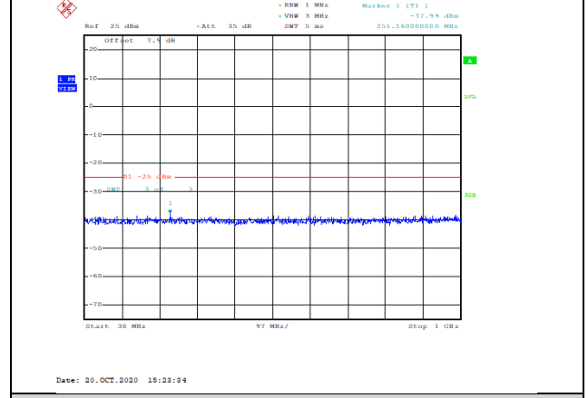
Band41-20MHz-QPSK-40140-1RB#0-Range1:30~1000MHz--37.99-PASS
