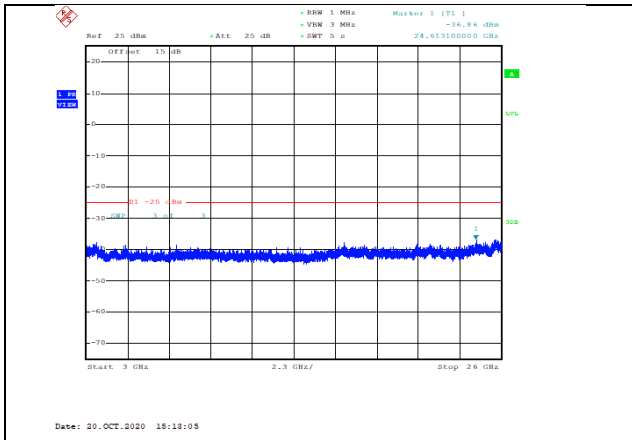
Band41-5MHz-QPSK-41215-1RB#0-Range3:3000~26000MHz--36.86-PASS
