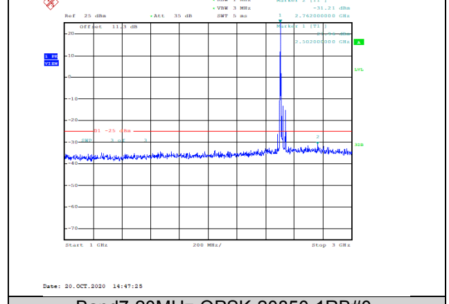
Band7-20MHz-QPSK-20850-1RB#0-Range2:1000~3000MHz--31.21-PASS
