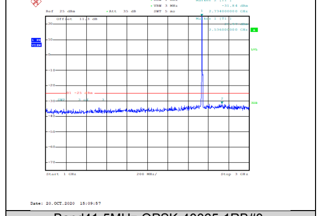
Band41-5MHz-QPSK-40065-1RB#0-Range2:1000~3000MHz--31.84-PASS
