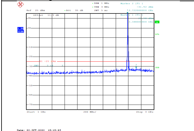
Band41-10MHz-QPSK-40590-1RB#0-Range2:1000~3000MHz--31.92-PASS
