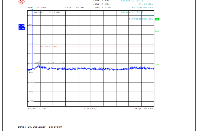
Band66-3MHz-QPSK-131987-1RB#0-Range2:1000~20000MHz--31.93-PASS
