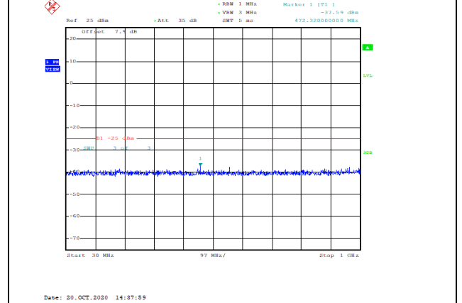
Band7-10MHz-QPSK-20800-1RB#0-Range1:30~1000MHz--37.59-PASS
