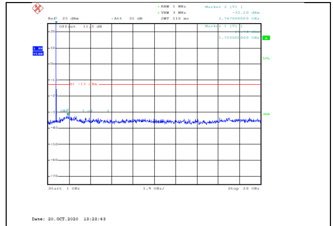
Band4-20MHz-QPSK-20300-1RB#0-Range2:1000~20000MHz--32.2-PASS
