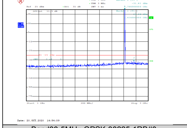
Band38-5MHz-QPSK-38225-1RB#0-Range2:1000~3000MHz--31.41-PASS
