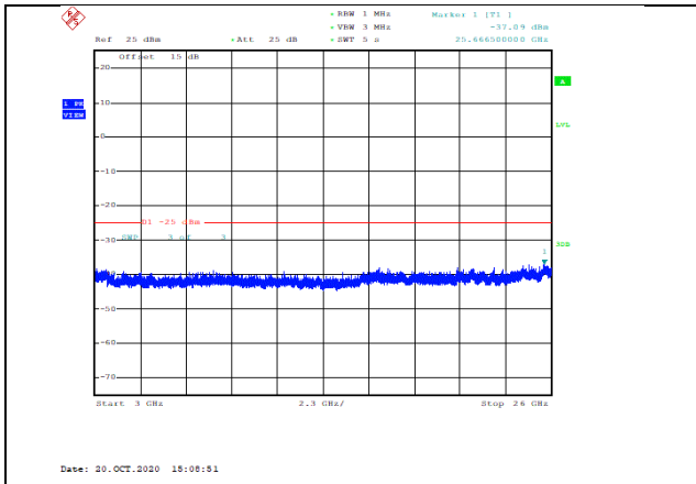
Band38-20MHz-QPSK-38150-1RB#0-Range3:3000~2600MHz--37.09-PASS
