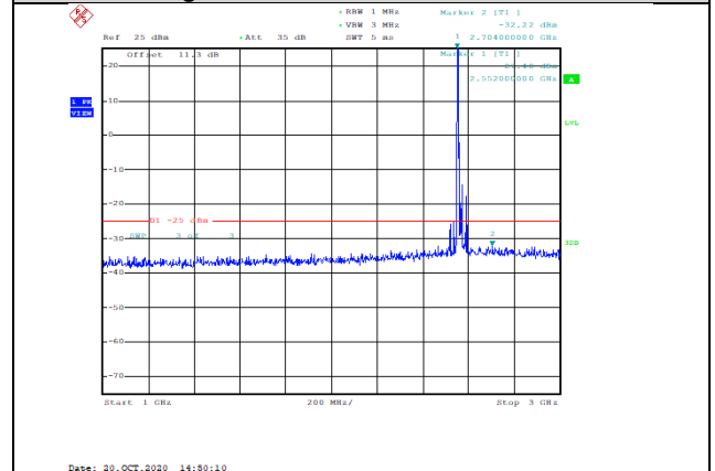
Band7-20MHz-QPSK-21350-1RB#0-Range2:1000~3000MHz--32.22-PASS
