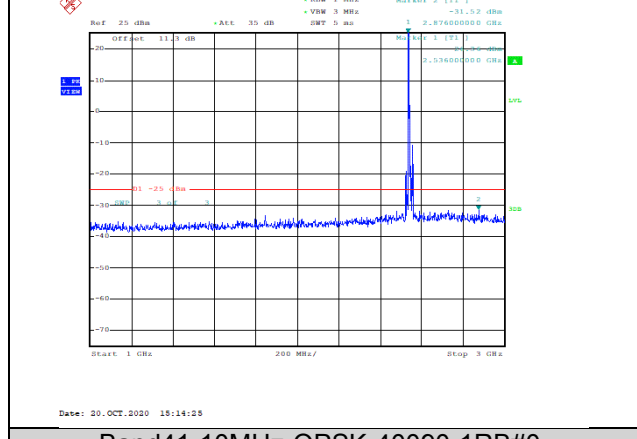
Band41-10MHz-QPSK-40090-1RB#0-Range2:1000~3000MHz--31.52-PASS
