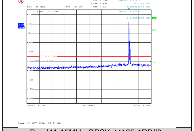
Band41-15MHz-QPSK-41165-1RB#0-Range2:1000~3000MHz--31.66-PASS
