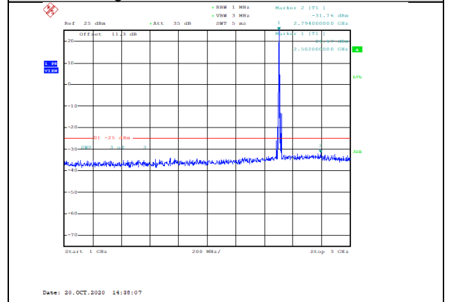
Band7-10MHz-QPSK-20800-1RB#0-Range2:1000~3000MHz--31.76-PASS
