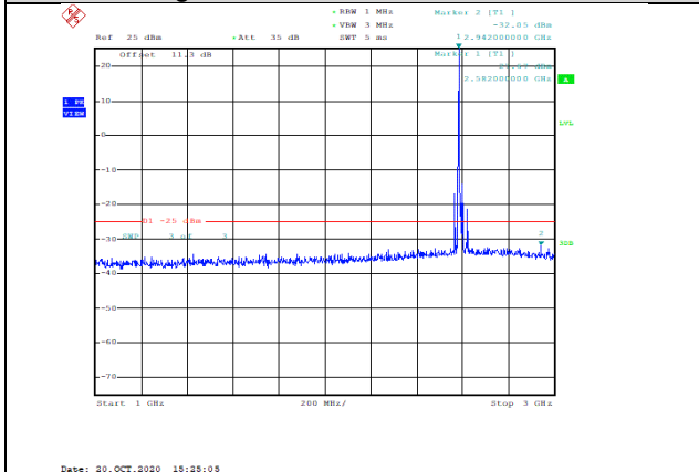
Band41-20MHz-QPSK-40590-1RB#0-Range2:1000~3000MHz--32.05-PASS
