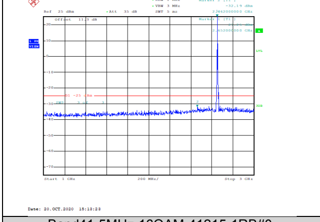
Band41-5MHz-16QAM-41215-1RB#0-Range2:1000~3000MHz--32.19-PASS
