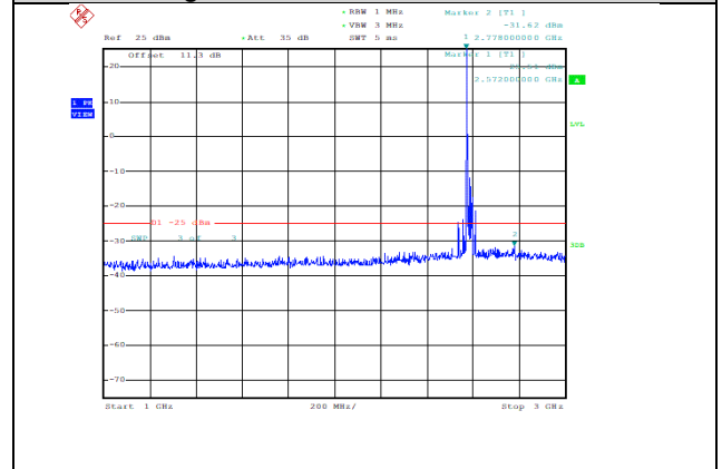
Band38-20MHz-QPSK-37850-1RB#0-Range2:1000~3000MHz--31.62-PASS
