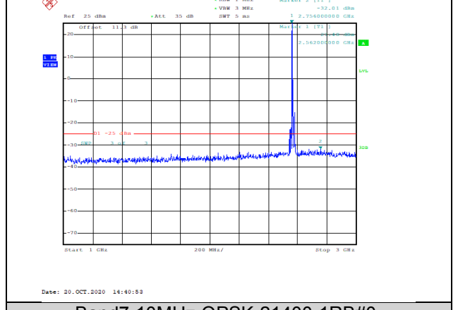
Band7-10MHz-QPSK-21400-1RB#0-Range2:1000~3000MHz--32.01-PASS
