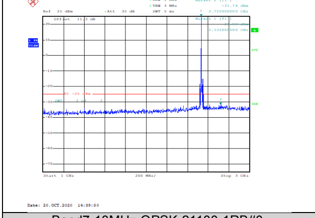
Band7-10MHz-QPSK-21100-1RB#0-Range2:1000~3000MHz--31.74-PASS
