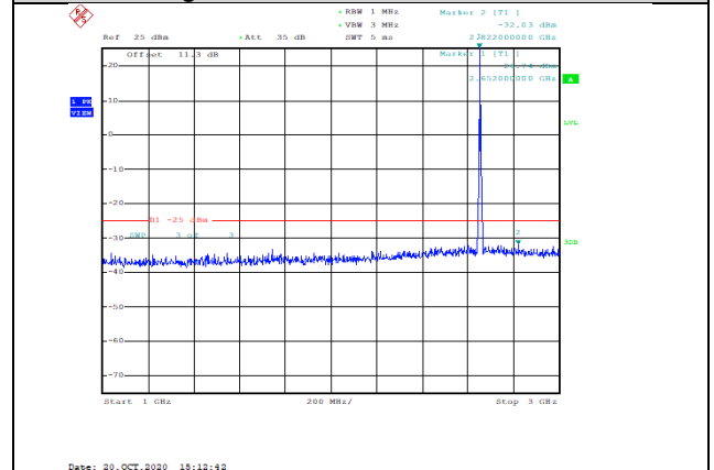
Band41-5MHz-QPSK-41215-1RB#0-Range2:1000~3000MHz--32.03-PASS
