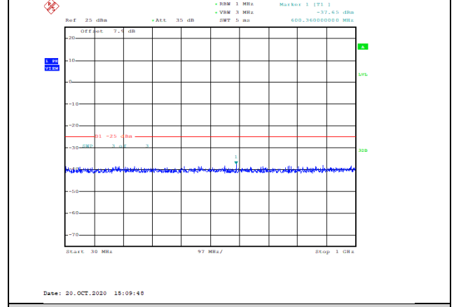
Band41-5MHz-QPSK-40065-1RB#0-Range1:30~1000MHz--37.65-PASS
