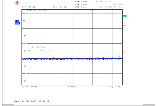
Band41-15MHz-QPSK-41165-1RB#0-Range1:30~1000MHz--37.7-PASS
