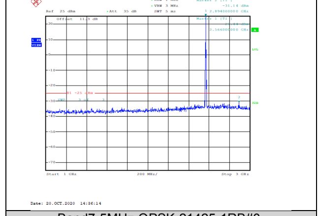
Band7-5MHz-QPSK-21425-1RB#0-Range2:1000~3000MHz--31.14-PASS
