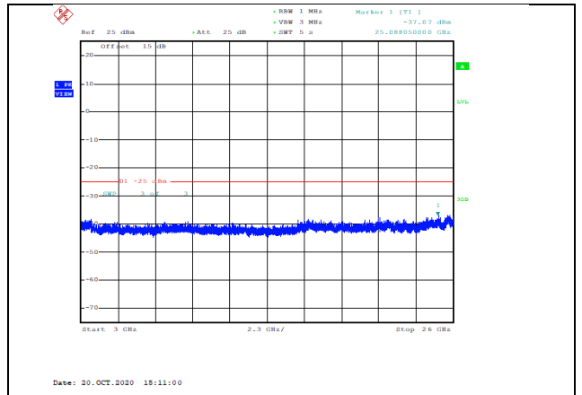
Band41-5MHz-16QAM-40065-1RB#0-Range3:3000~26000MHz--37.07-PASS
