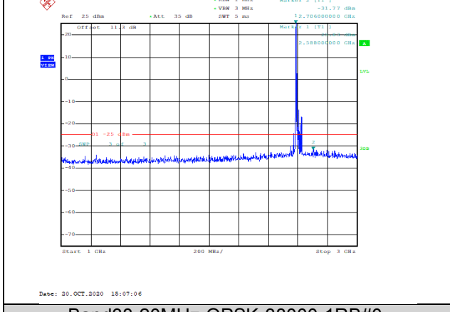
Band38-20MHz-QPSK-38000-1RB#0-Range2:1000~3000MHz--31.77-PASS
