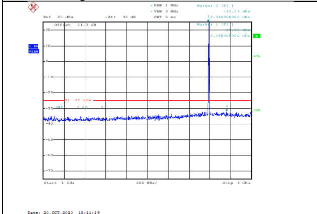
Band41-5MHz-QPSK-40590-1RB#0-Range2:1000~3000MHz--32.13-PASS
