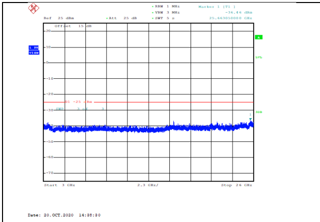
Band7-10MHz-QPSK-20800-1RB#0-Range3:3000~26000MHz--36.46-PASS
