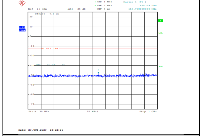
Band4-20MHz-QPSK-20050-1RB#0-Range1:30~1000MHz--38.09-PASS
