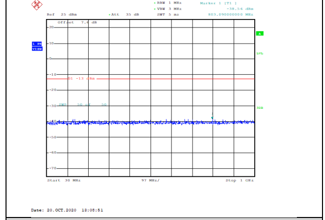
Band2-20MHz-QPSK-18700-1RB#0-Range1:30~1000MHz--38.56-PASS
