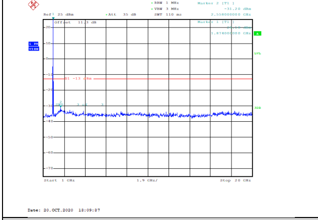
Band2-20MHz-QPSK-18900-1RB#0-Range2:1000~20000MHz--31.2-PASS
