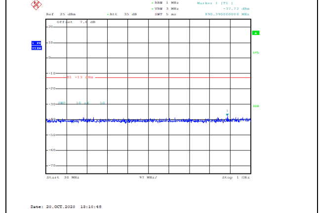
Band4-1.4MHz-QPSK-19957-1RB#0-Range1:30~1000MHz--37.72-PASS
