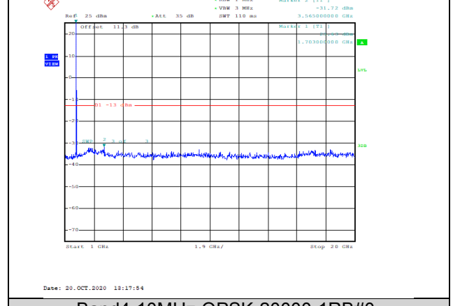
Band4-10MHz-QPSK-20000-1RB#0-Range2:1000~20000MHz--31.72-PASS
