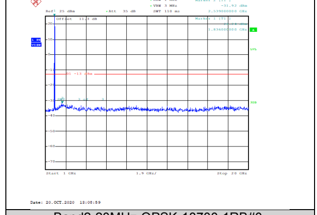
Band2-20MHz-QPSK-18700-1RB#0-Range2:1000~20000MHz--31.92-PASS
