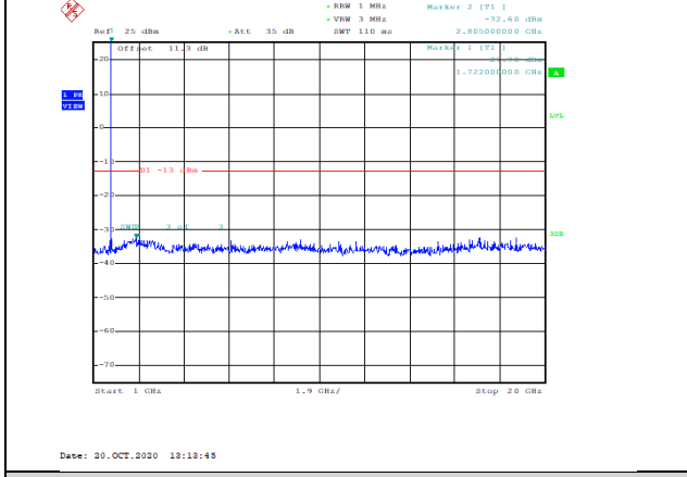
Band4-3MHz-QPSK-20175-1RB#0-Range2:1000~20000MHz--32.6-PASS
