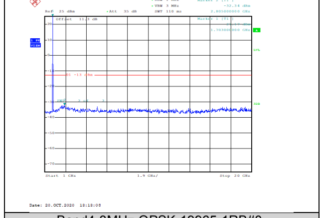
Band4-3MHz-QPSK-19965-1RB#0-Range2:1000~20000MHz--32.34-PASS
