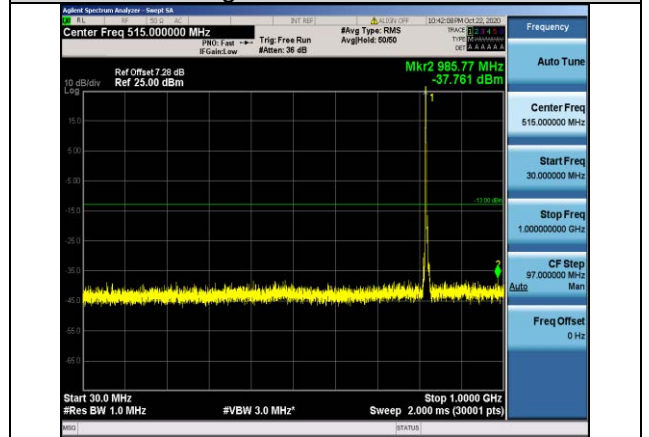
Band26-5MHz-QPSK-26765-1RB#0- Range1:30~1000MHz
