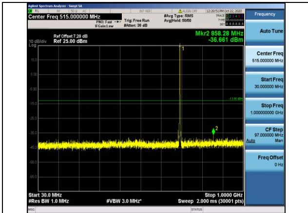
Band12-1.4MHz-QPSK-23017-1RB#0- Range1:30~1000MHz
