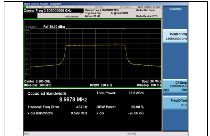
Band7-10MHz-QPSK-20800-50RB#0-8.9878
