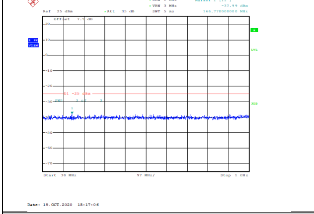
Band7-20MHz-QPSK-21100-1RB#0-Range1:30~1000MHz--37.99-PASS
