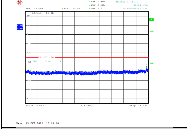
Band41-5MHz-QPSK-41215-1RB#0-Range3:3000~26000MHz--36.04-PASS
