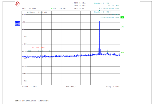
Band41-5MHz-QPSK-40590-1RB#0-Range2:1000~3000MHz--31.64-PASS
