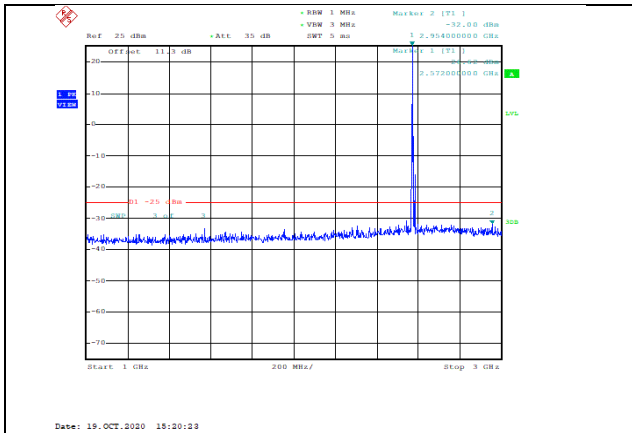
Band38-5MHz-QPSK-37775-1RB#0-Range2:1000~3000MHz--32-PASS
