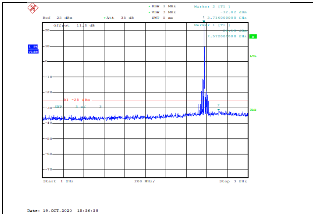
Band38-20MHz-QPSK-37850-1RB#0-Range2:1000~3000MHz--32.02-PASS
