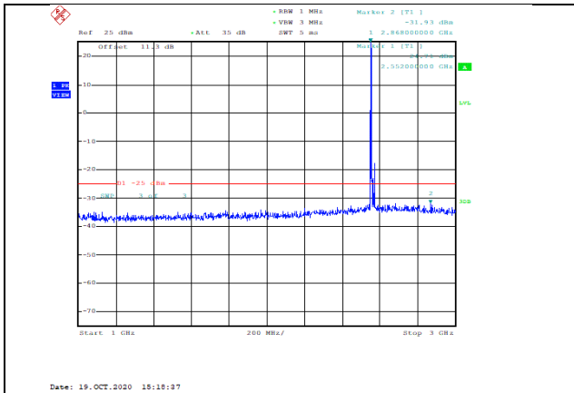
Band7-20MHz-QPSK-21350-1RB#0-Range2:1000~3000MHz--31.93-PASS
