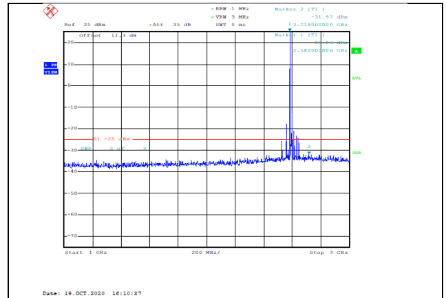
Band41-20MHz-QPSK-40590-1RB#0-Range2:1000~3000MHz--31.97-PASS
