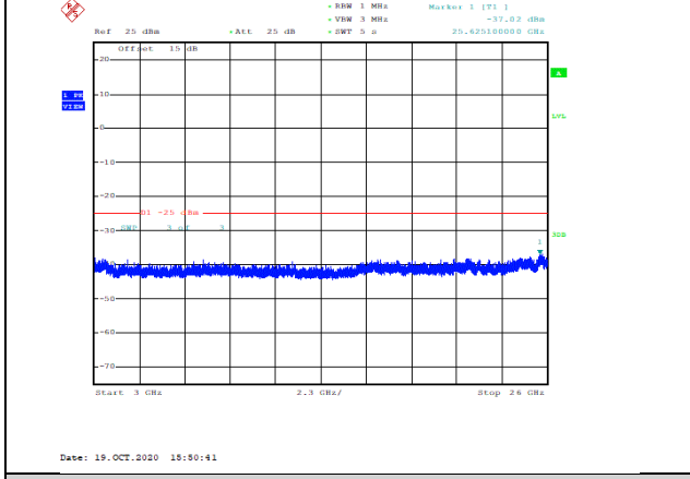
Band41-10MHz-QPSK-40090-1RB#0-Range3:3000~26000MHz--37.02-PASS
