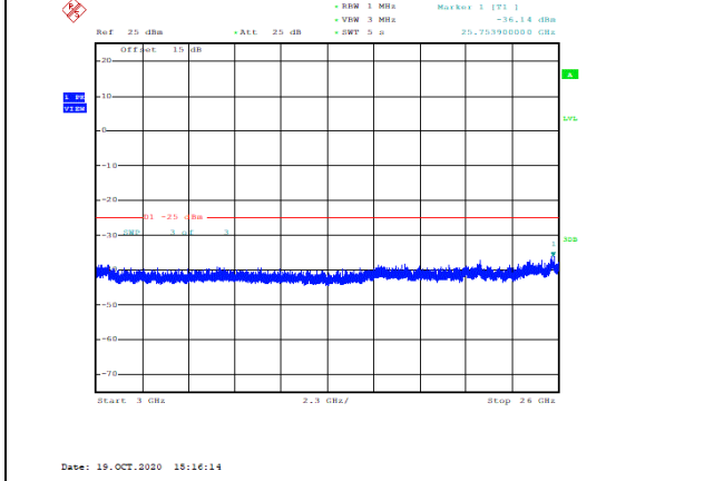
Band7-20MHz-QPSK-20850-1RB#0-Range3:3000~26000MHz--36.14-PASS
