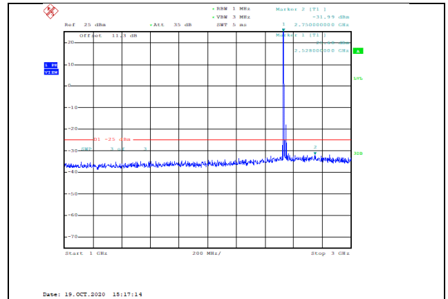
Band7-20MHz-QPSK-21100-1RB#0-Range2:1000~3000MHz--31.99-PASS
