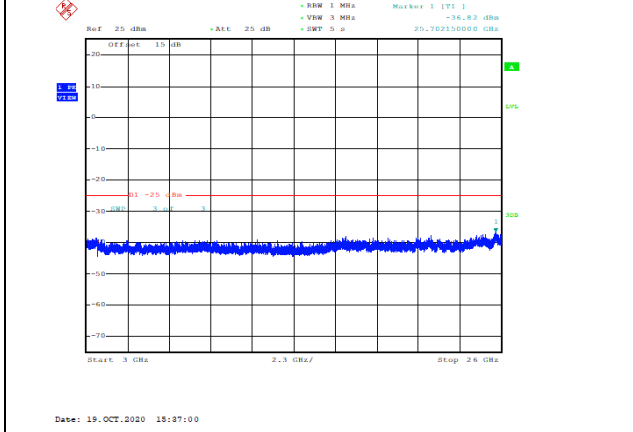
Band38-20MHz-QPSK-37850-1RB#0-Range3:3000~26000MHz--36.82-PASS
