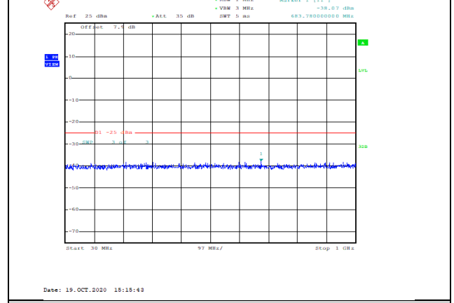
Band7-20MHz-QPSK-20850-1RB#0-Range1:30~1000MHz--38.07-PASS
