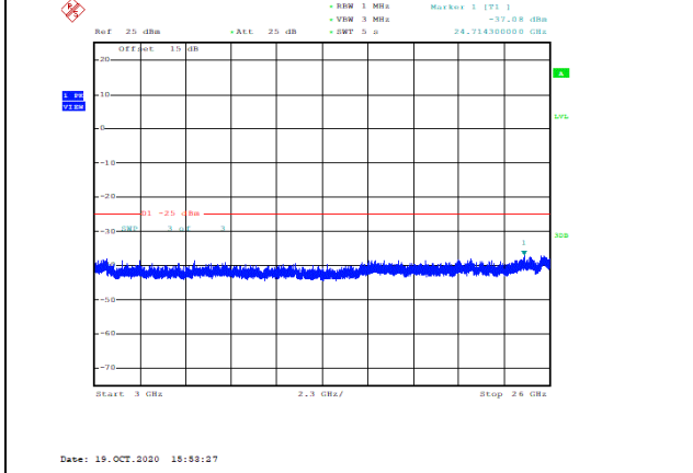
Band41-10MHz-QPSK-41190-1RB#0-Range3:3000~26000MHz--37.08-PASS
