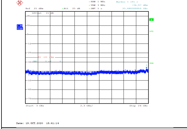
Band41-5MHz-QPSK-40065-1RB#0-Range3:3000~26000MHz--36.97-PASS
