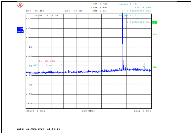
Band41-10MHz-QPSK-40090-1RB#0-Range2:1000~3000MHz--31.56-PASS
