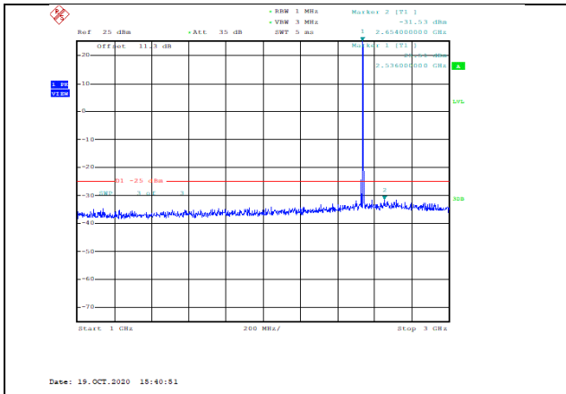
Band41-5MHz-QPSK-40065-1RB#0-Range2:1000~3000MHz--31.53-PASS
