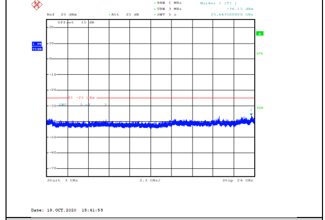
Band41-5MHz-16QAM-40065-1RB#0-Range3:3000~26000MHz--36.15-PASS
