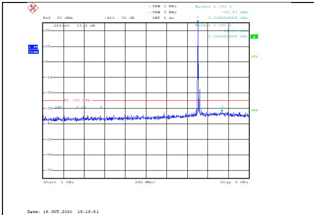
Band7-20MHz-QPSK-20850-1RB#0-Range2:1000~3000MHz--32.37-PASS
