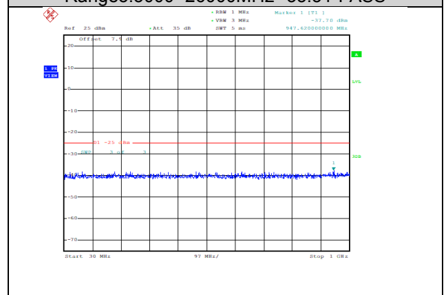
Band41-15MHz-QPSK-41165-1RB#0-Range1:30~1000MHz--37.7-PASS
