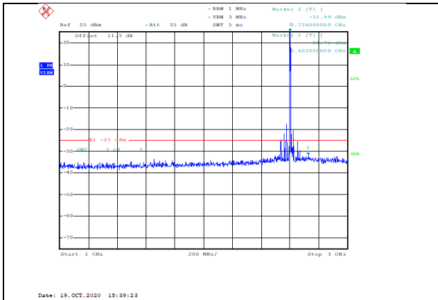
Band38-20MHz-QPSK-38150-1RB#0-Range2:1000~3000MHz--31.99-PASS
