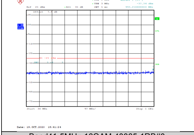
Band41-5MHz-16QAM-40065-1RB#0-Range1:30~1000MHz--37.34-PASS
