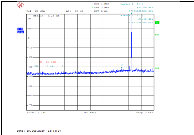
Band41-5MHz-QPSK-41215-1RB#0-Range2:1000~3000MHz--31.46-PASS
