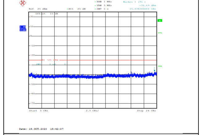
Band41-5MHz-QPSK-40590-1RB#0-Range3:3000~26000MHz--36.69-PASS
