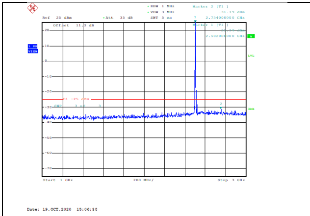
Band7-10MHz-QPSK-20800-1RB#0-Range2:1000~3000MHz--31.39-PASS
