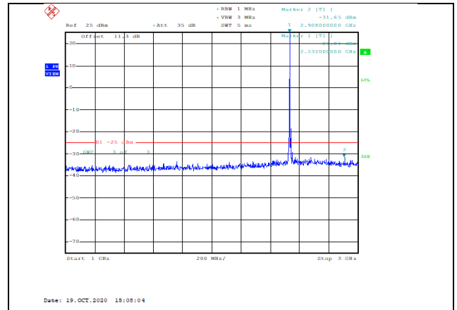
Band7-10MHz-QPSK-21100-1RB#0-Range2:1000~3000MHz--31.65-PASS
