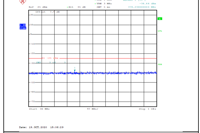
Band7-10MHz-QPSK-20800-1RB#0-Range1:30~1000MHz--38.44-PASS
