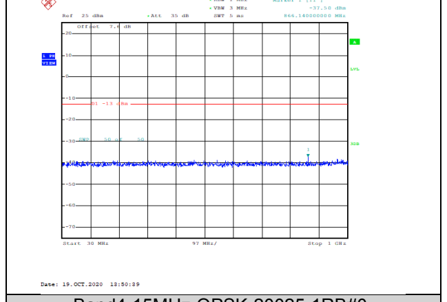
Band4-15MHz-QPSK-20025-1RB#0-Range1:30~1000MHz--37.5-PASS
