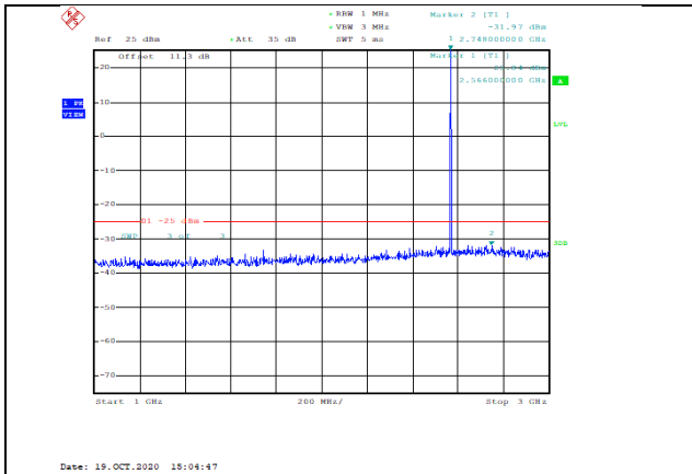
Band7-5MHz-QPSK-21425-1RB#0-Range2:1000~3000MHz--31.97-PASS
