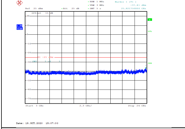
Band7-10MHz-QPSK-20800-1RB#0-Range3:3000~26000MHz--37.41-PASS
