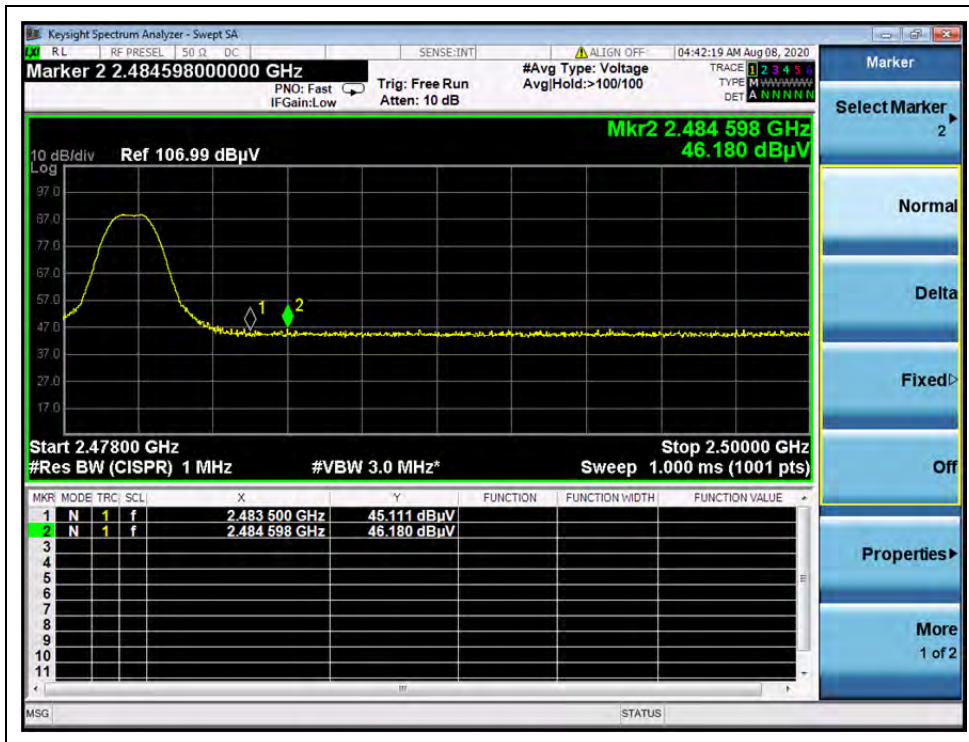
(AVERAGE, Channel 39)
