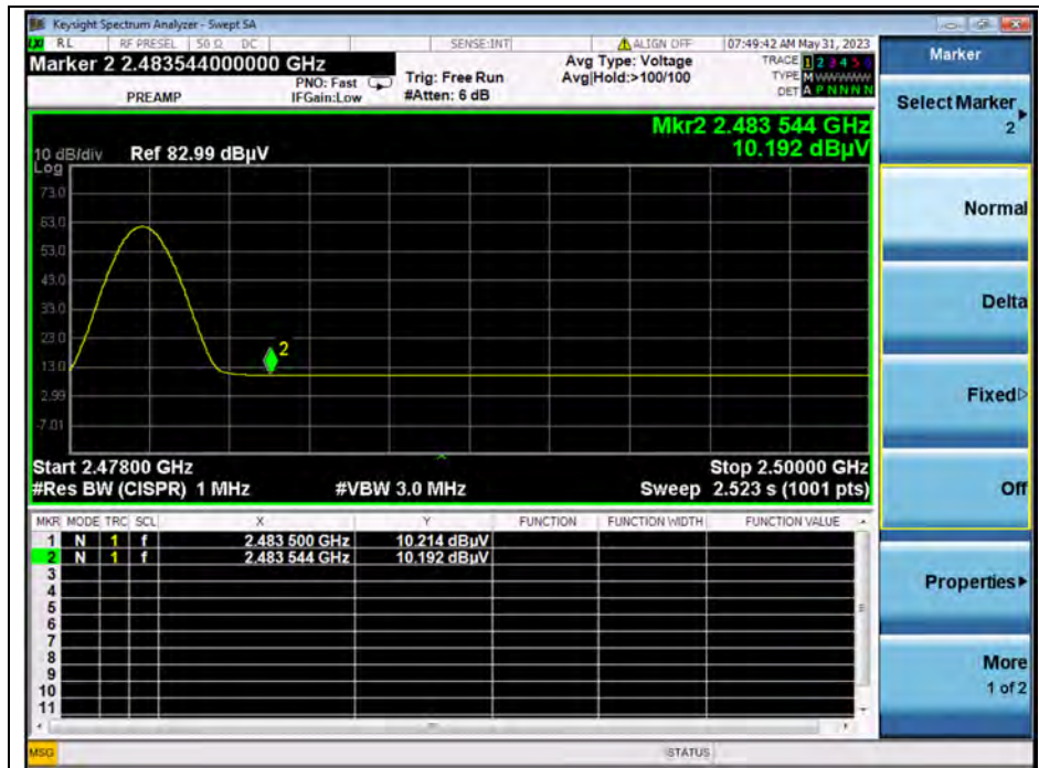
(AVERAGE, Channel 39)
