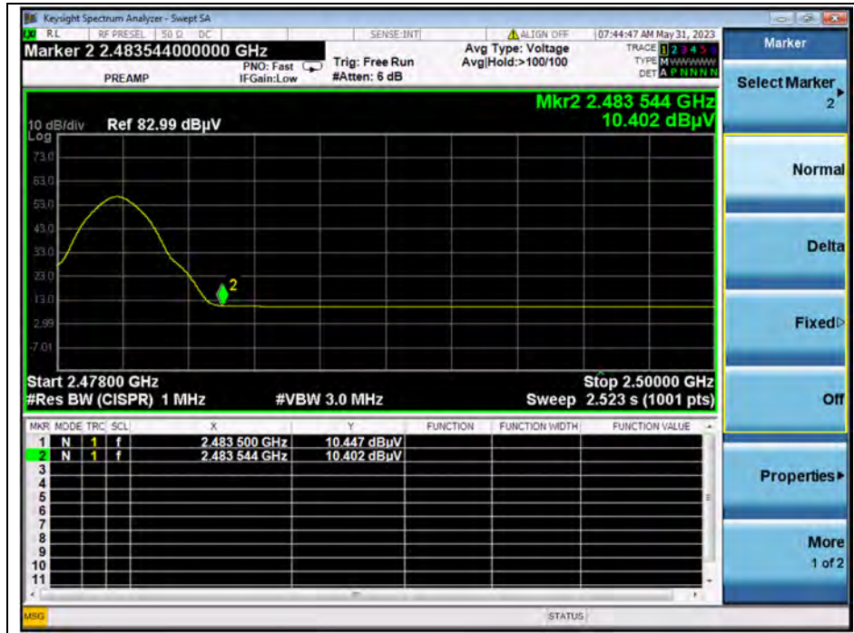
(AVERAGE, Channel 39)
