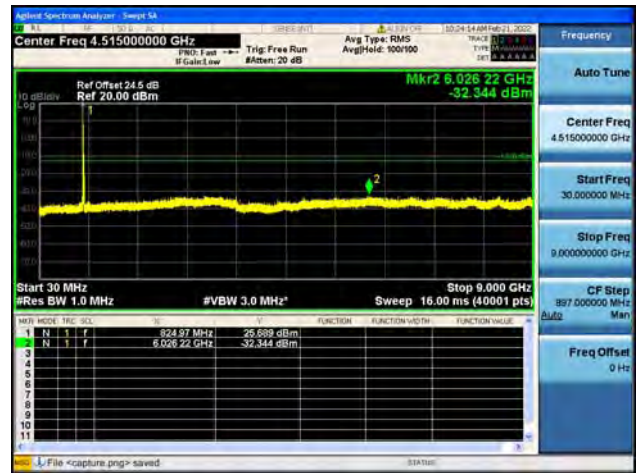
Band26 / 15MHz / Mid CH / QPSK
