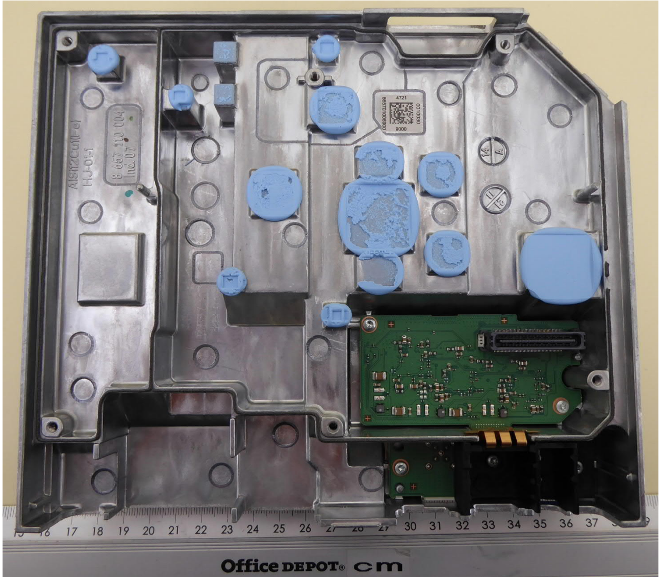
EUT open 3
