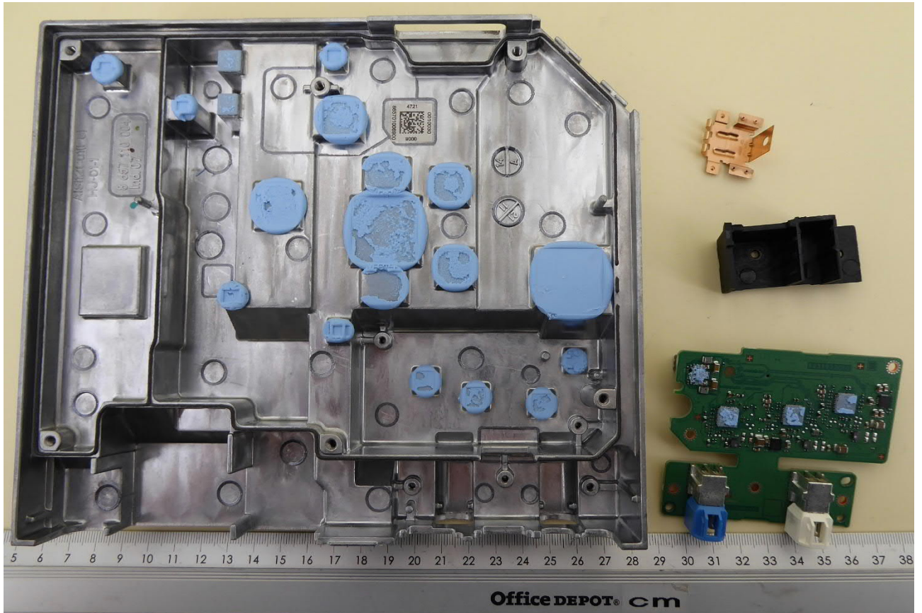
EUT open 4
