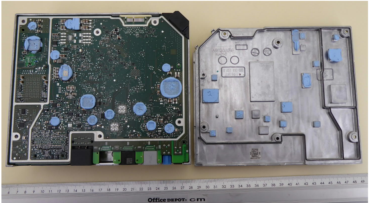
EUT open 1
