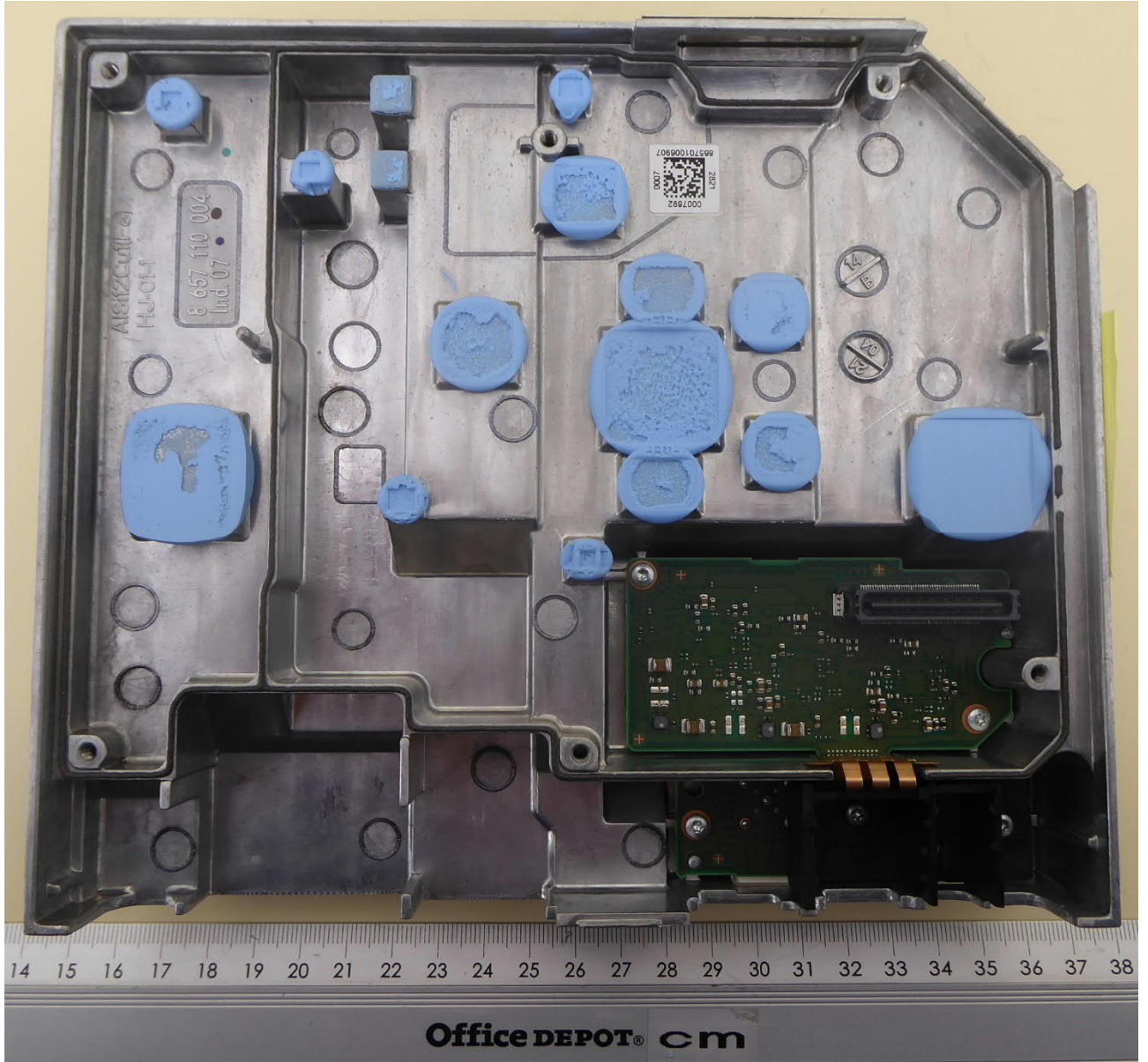
EUT open 3
