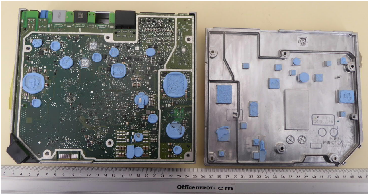
EUT open 1
