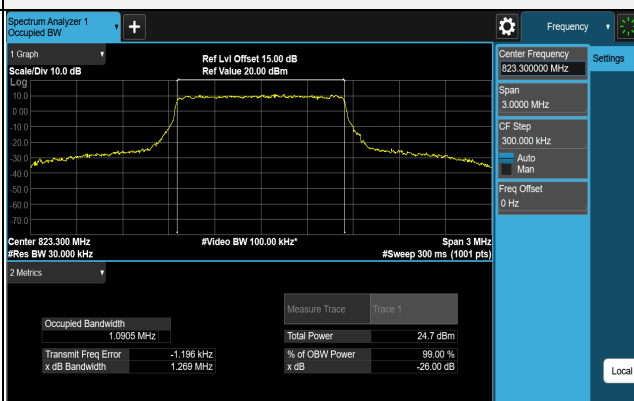
QPSK CH 26783 (823.3MHz)
