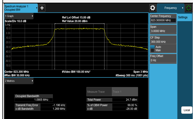
QPSK CH 26783 (823.3MHz)
