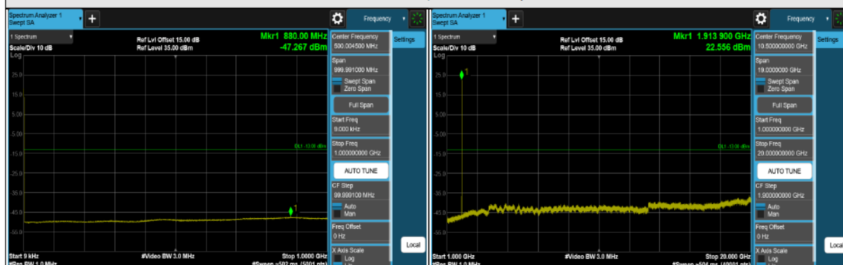
CH 26683 (1914.3MHz)
