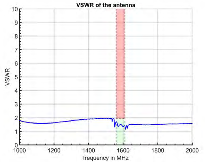
Output VSWR
