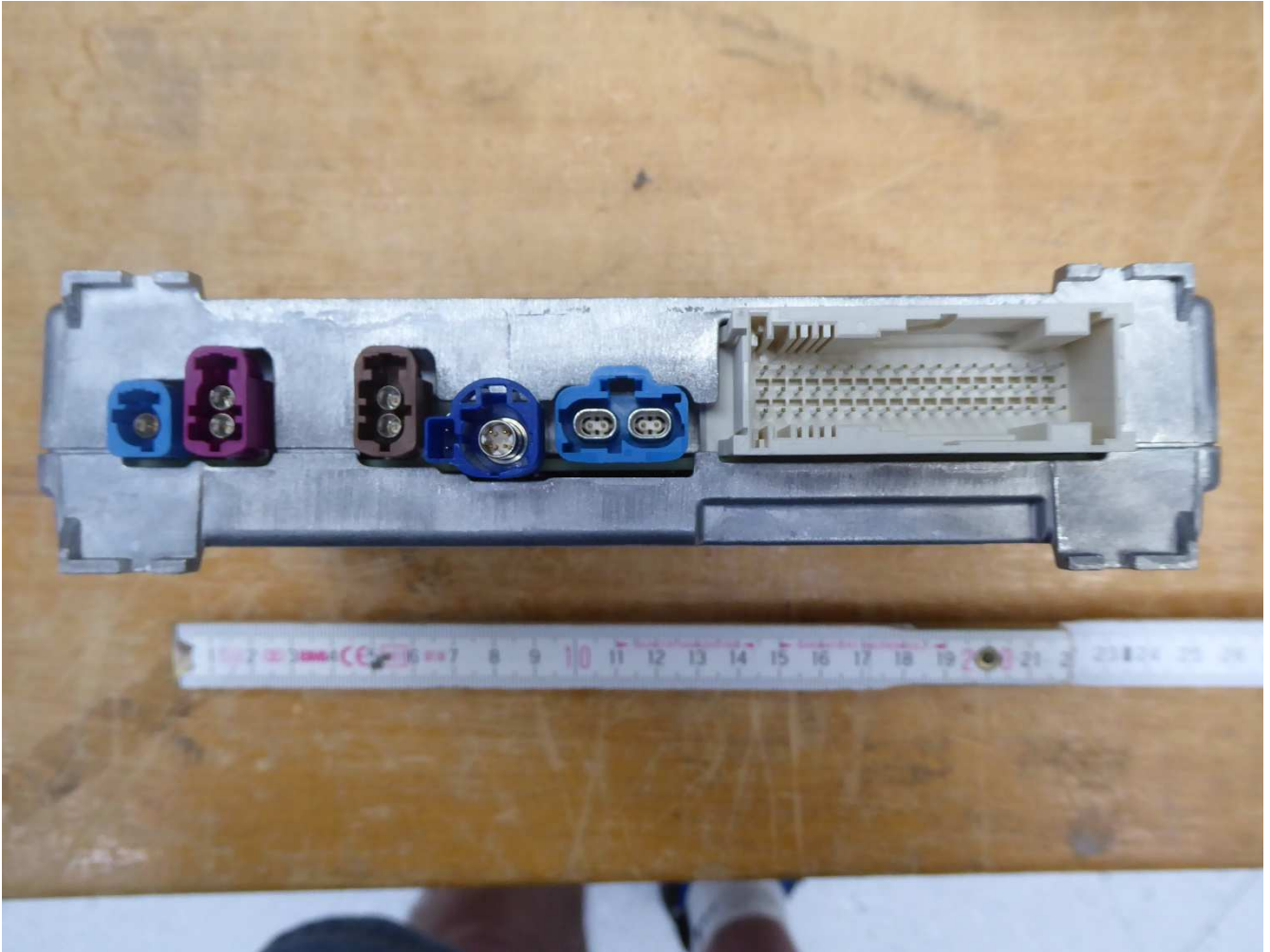
EUT Connectors
