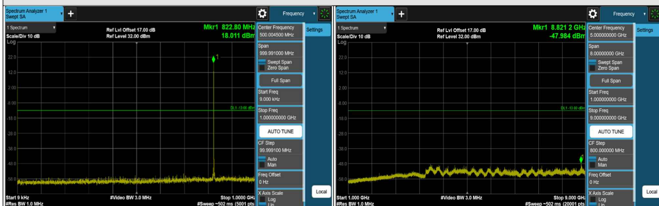
CH 26783 (823.3MHz)
