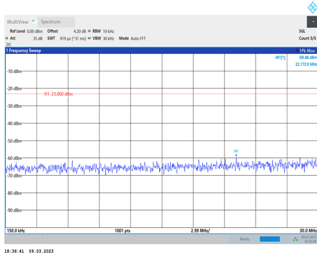
Band4-20MHz-QPSK-20050-1RB#0-Range2:0.15~30MHz
