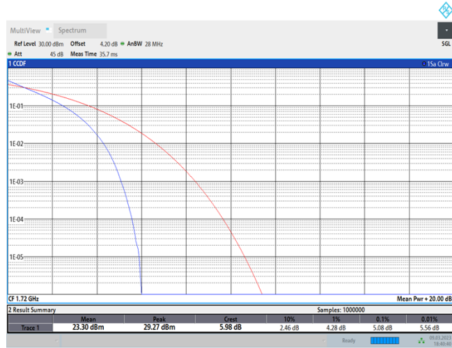
Band4-20MHz-QPSK-20050-100RB#0
