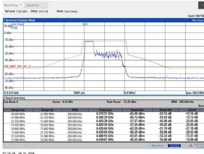
11AX20MIMO_Ant2_6415_106Tone_RU53
