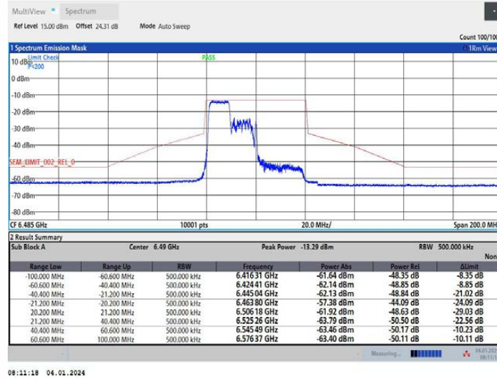
11AX40MIMO_Ant2_6485_242Tone_RU61
