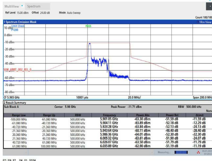
11AX40MIMO_Ant1_5965_52Tone_RU37
