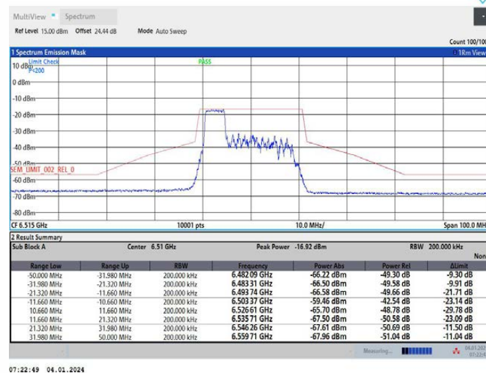
11AX20MIMO_Ant1_6515_106Tone_RU53
