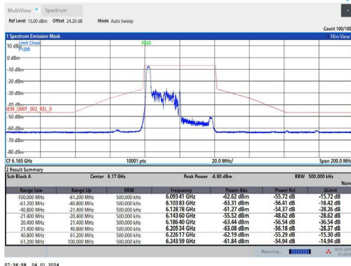
11AX40MIMO_Ant2_6165_52Tone_RU37
