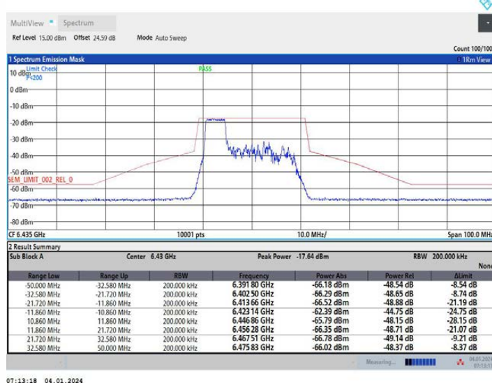
11AX20MIMO_Ant1_6435_106Tone_RU53
