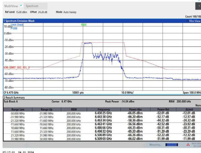
11AX20MIMO_Ant2_6475_106Tone_RU53
