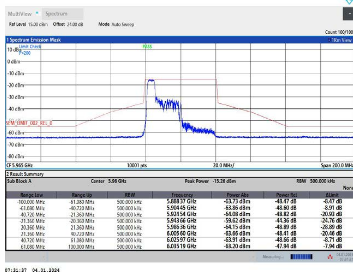
11AX40MIMO_Ant1_5965_106Tone_RU53
