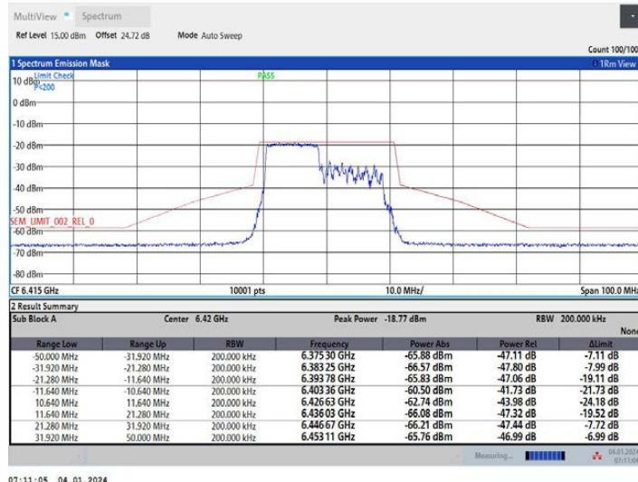
11AX20MIMO_Ant2_6415_26Tone_RU0
