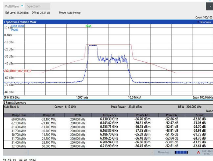
11AX20MIMO_Ant2_6175_106Tone_RU53
