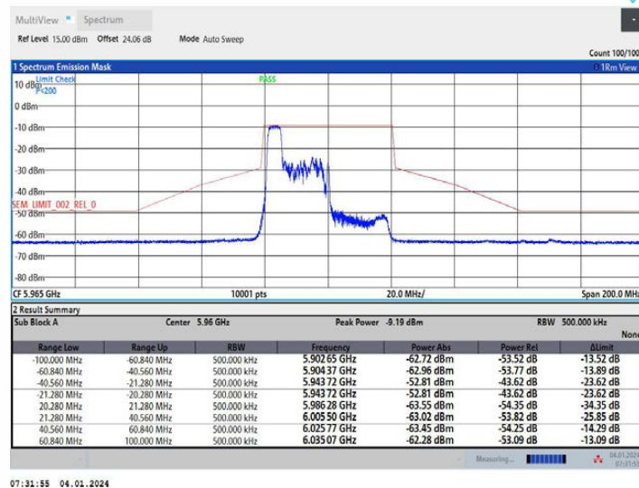
11AX40MIMO_Ant2_5965_106Tone_RU53
