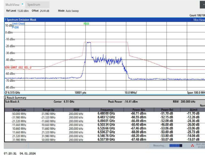
11AX20MIMO_Ant1_6515_52Tone_RU37
