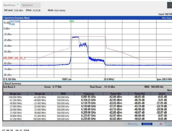
11AX40MIMO_Ant2_6165_242Tone_RU61
