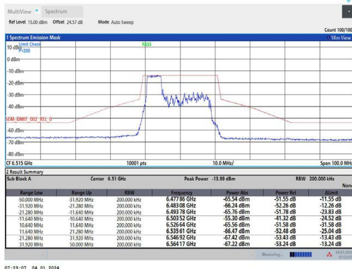
11AX20MIMO_Ant2_6515_106Tone_RU53
