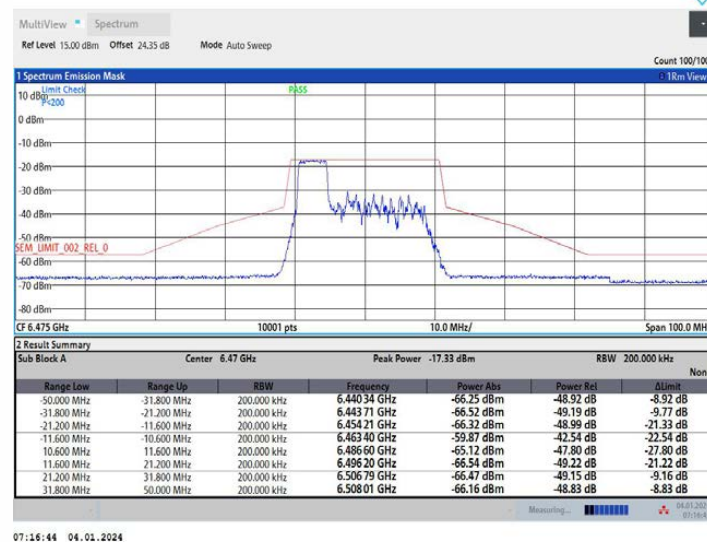
11AX20MIMO_Ant1_6475_106Tone_RU53
