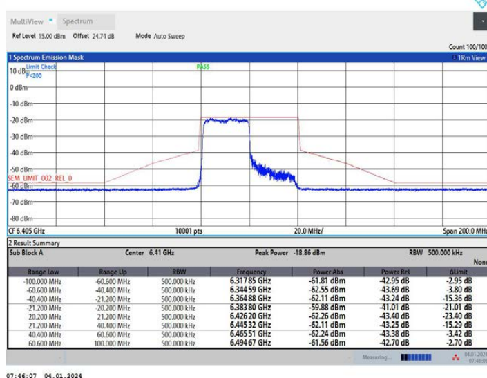
11AX40MIMO_Ant2_6405_26Tone_RU0
