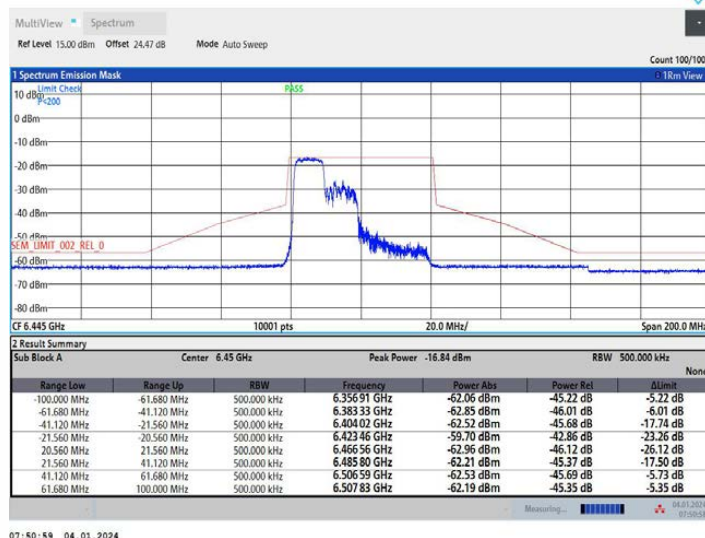
11AX40MIMO_Ant1_6445_242Tone_RU61
