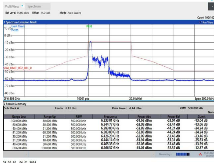
11AX40MIMO_Ant1_6405_52Tone_RU37
