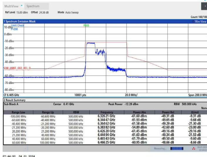
11AX40MIMO_Ant2_6405_242Tone_RU61
