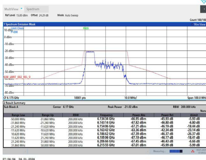
11AX20MIMO_Ant1_6175_106Tone_RU53
