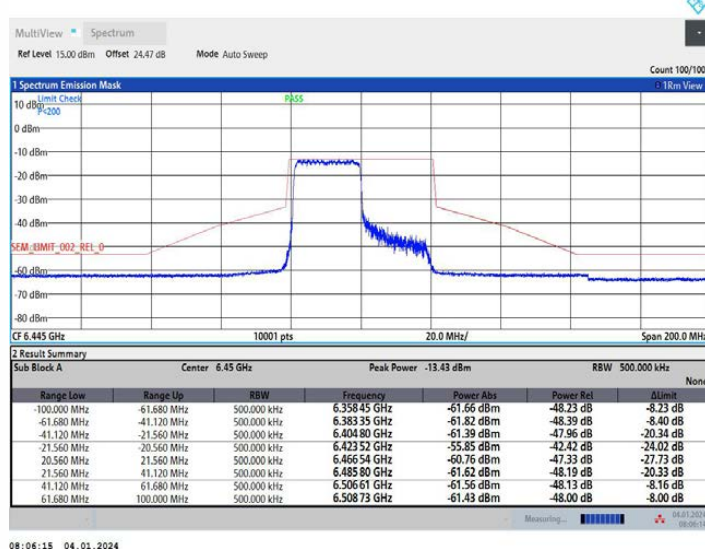
11AX40MIMO_Ant2_6445_26Tone_RU0
