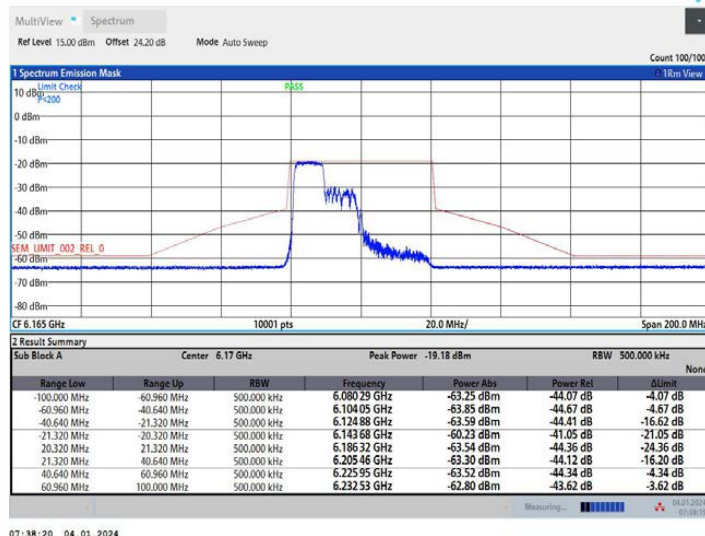
11AX40MIMO_Ant1_6165_242Tone_RU61
