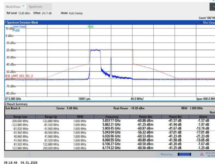
11AX80MIMO_Ant1_5985_484Tone_RU65
