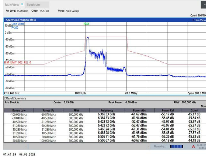
11AX40MIMO_Ant2_6445_52Tone_RU37
