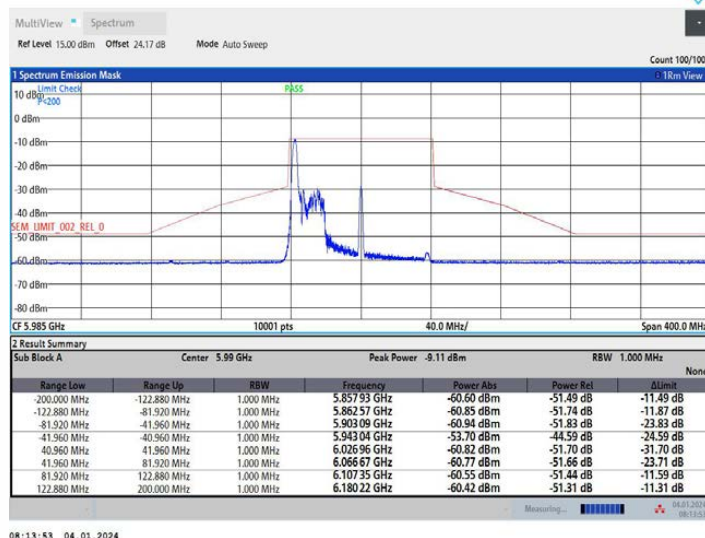
11AX80MIMO_Ant1_5985_52Tone_RU37
