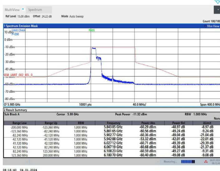
11AX80MIMO_Ant2_5985_242Tone_RU61
