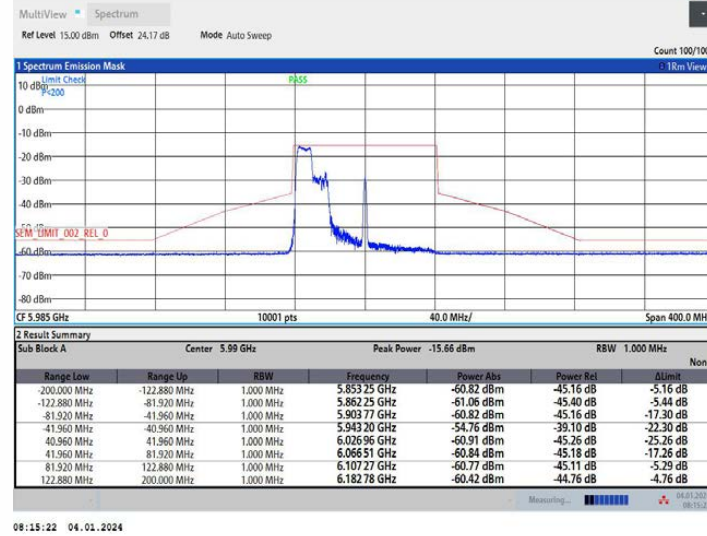
11AX80MIMO_Ant1_5985_242Tone_RU61
