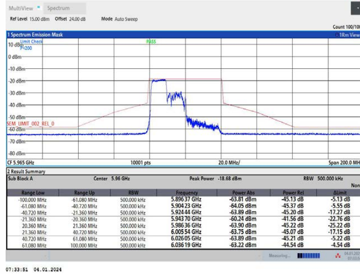
11AX40MIMO_Ant1_5965_242Tone_RU61
