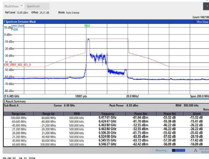
11AX40MIMO_Ant2_6485_52Tone_RU37
