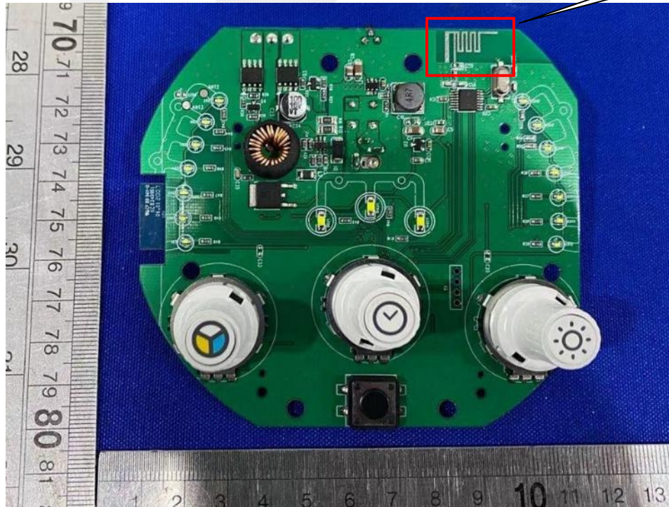
2.4G ANT
