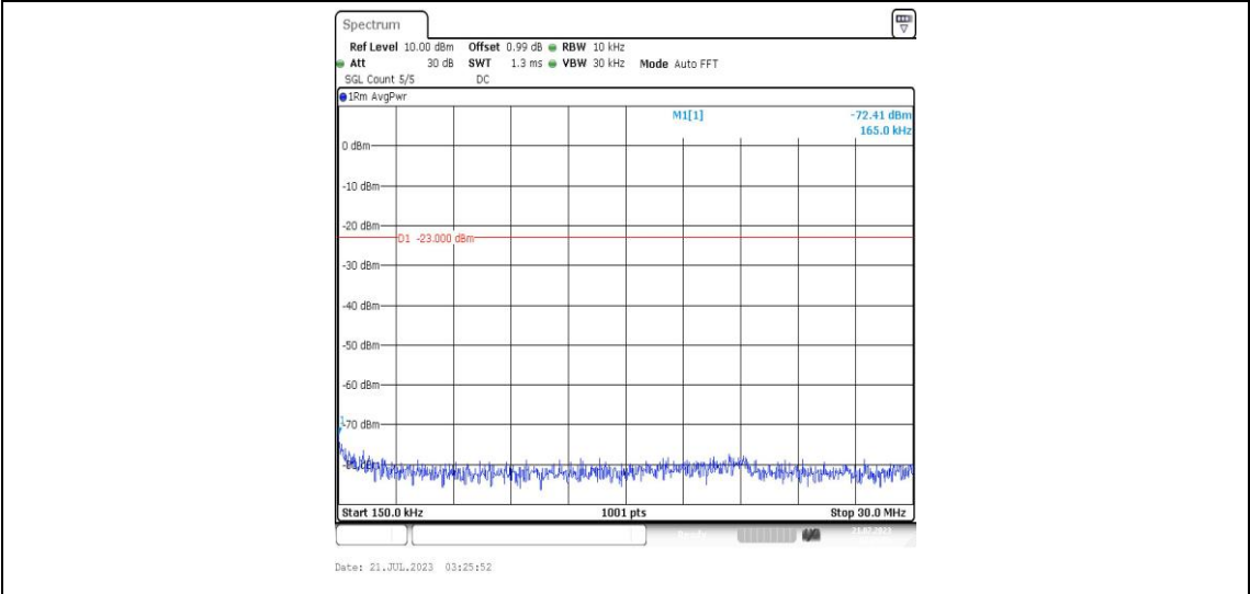
Band25-20MHz-16QAM-26590-1RB#0-Range2:0.15~30MHz-PASS
