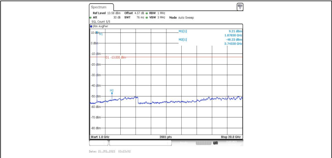
Band25-20MHz-QPSK-26365-1RB#0-Range4:1000~20000MHz-PASS
