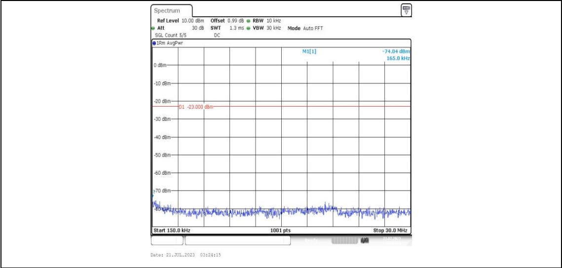
Band25-20MHz-16QAM-26365-1RB#0-Range2:0.15~30MHz-PASS
