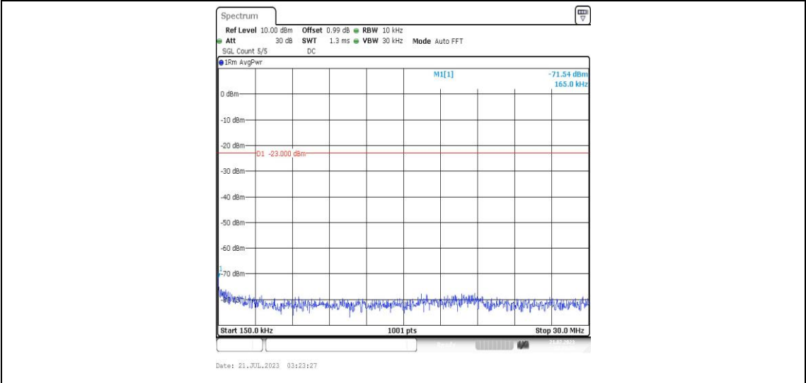
Band25-20MHz-QPSK-26365-1RB#0-Range2:0.15~30MHz-PASS
