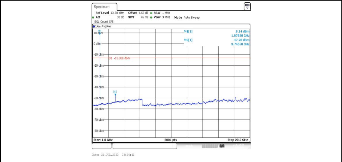
Band25-20MHz-16QAM-26365-1RB#0-Range4:1000~20000MHz-PASS
