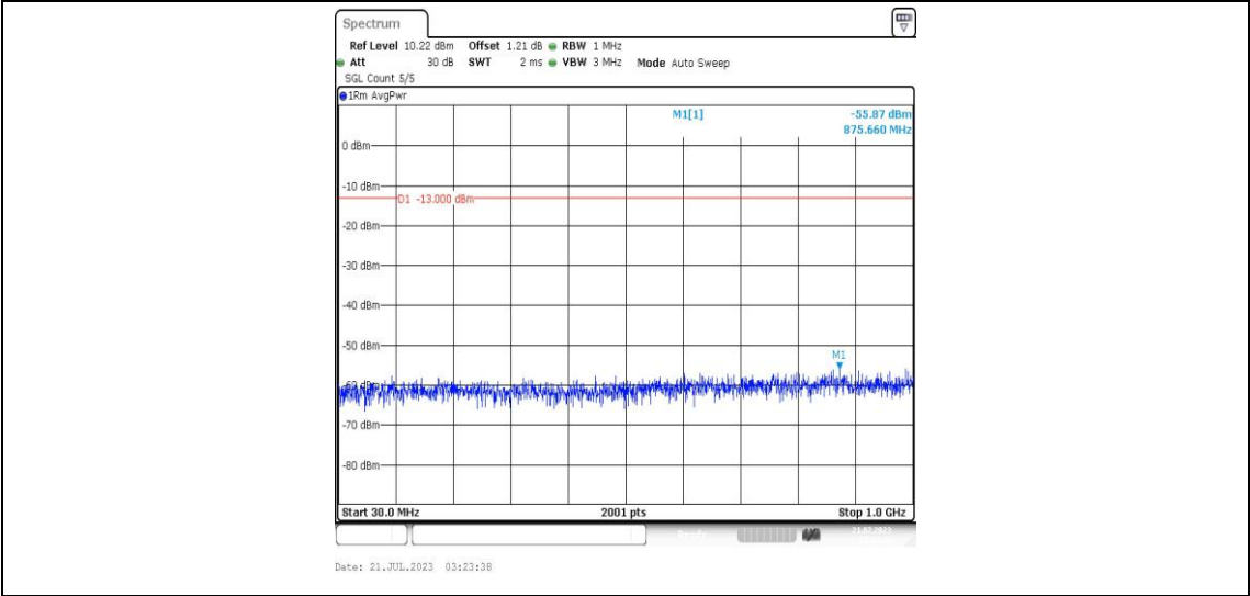
Band25-20MHz-QPSK-26365-1RB#0-Range3:30~1000MHz-PASS
