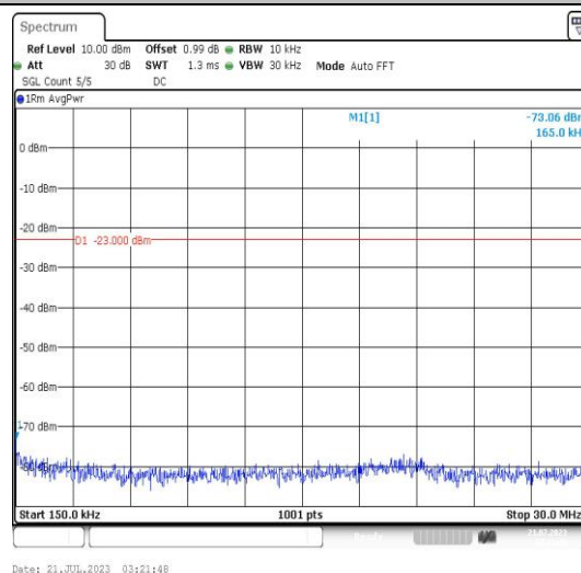
Band25-20MHz-QPSK-26140-1RB#0-Range2:0.15~30MHz-PASS
