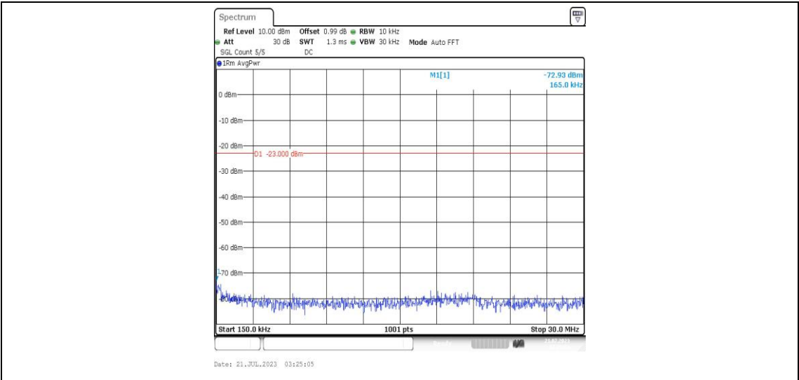
Band25-20MHz-QPSK-26590-1RB#0-Range2:0.15~30MHz-PASS
