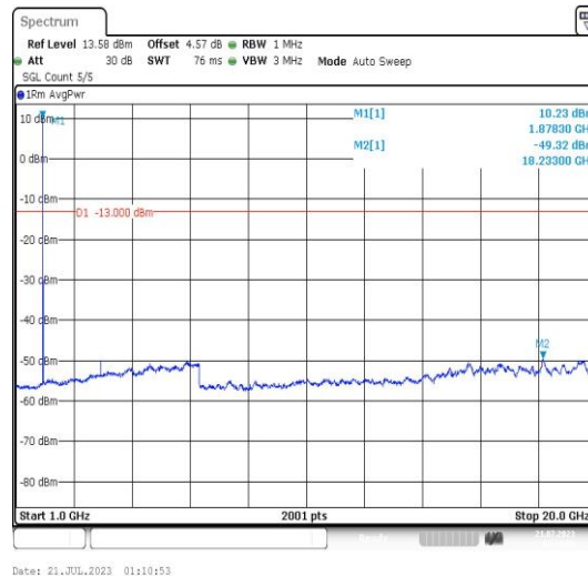
Band25-3MHz-QPSK-26365-1RB#0-Range4:1000~20000MHz-PASS
