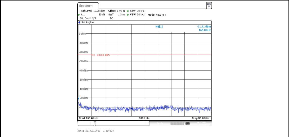
Band25-3MHz-QPSK-26365-1RB#0-Range2:0.15~30MHz-PASS
