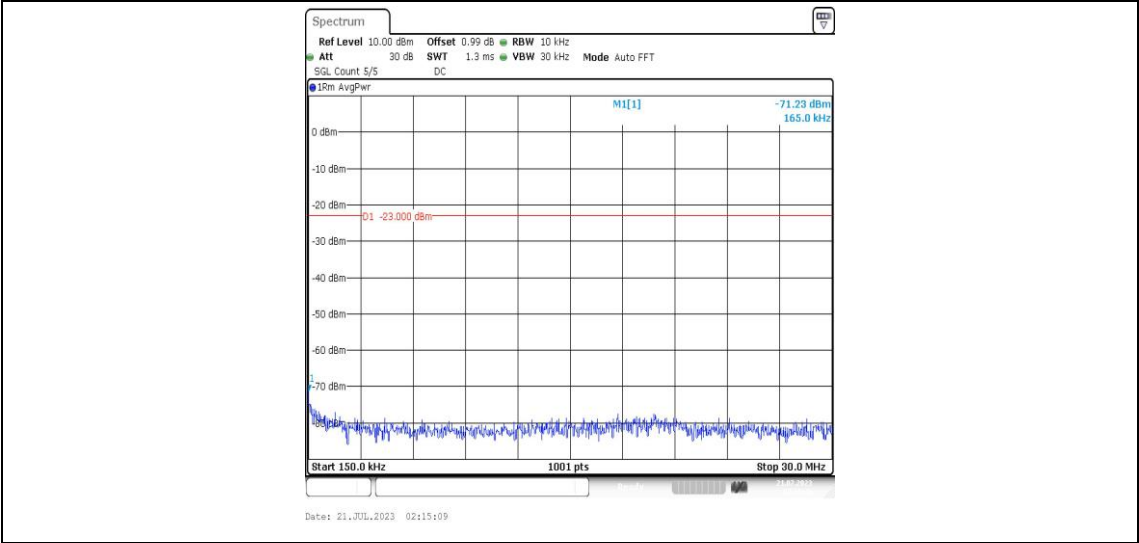
Band25-10MHz-QPSK-26090-1RB#0-Range2:0.15~30MHz-PASS
