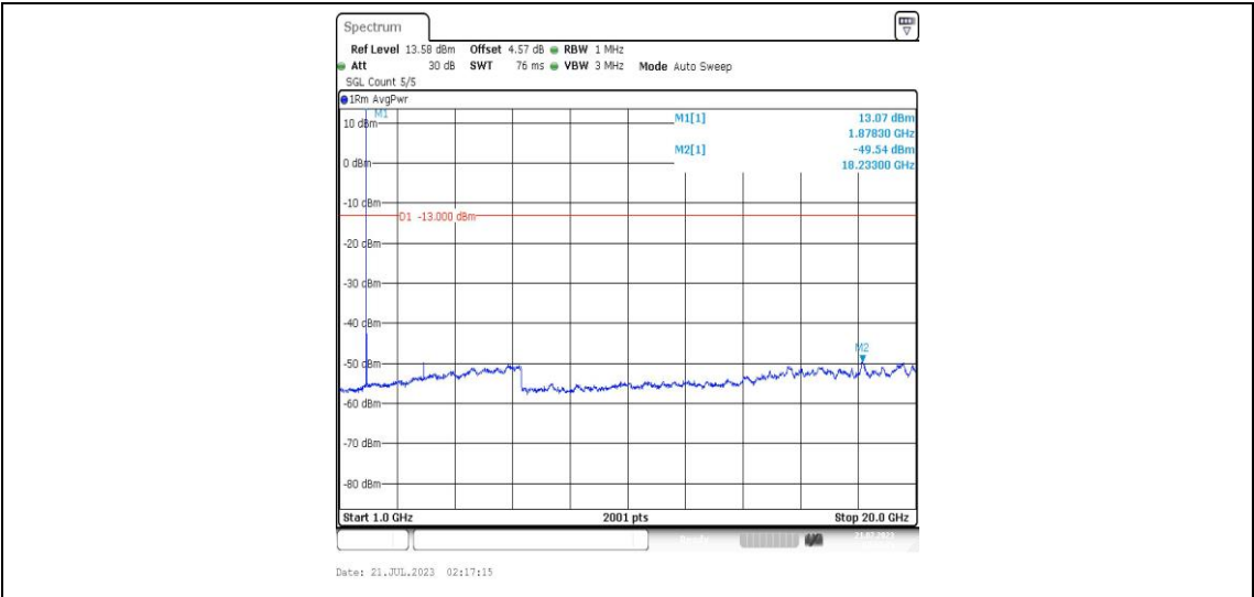
Band25-10MHz-QPSK-26365-1RB#0-Range4:1000~20000MHz-PASS
