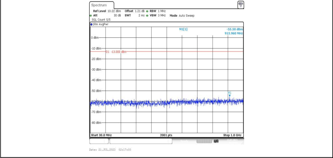
Band25-10MHz-QPSK-26365-1RB#0-Range3:30~1000MHz-PASS
