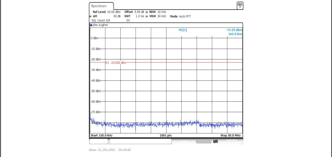
Band25-10MHz-QPSK-26365-1RB#0-Range2:0.15~30MHz-PASS
