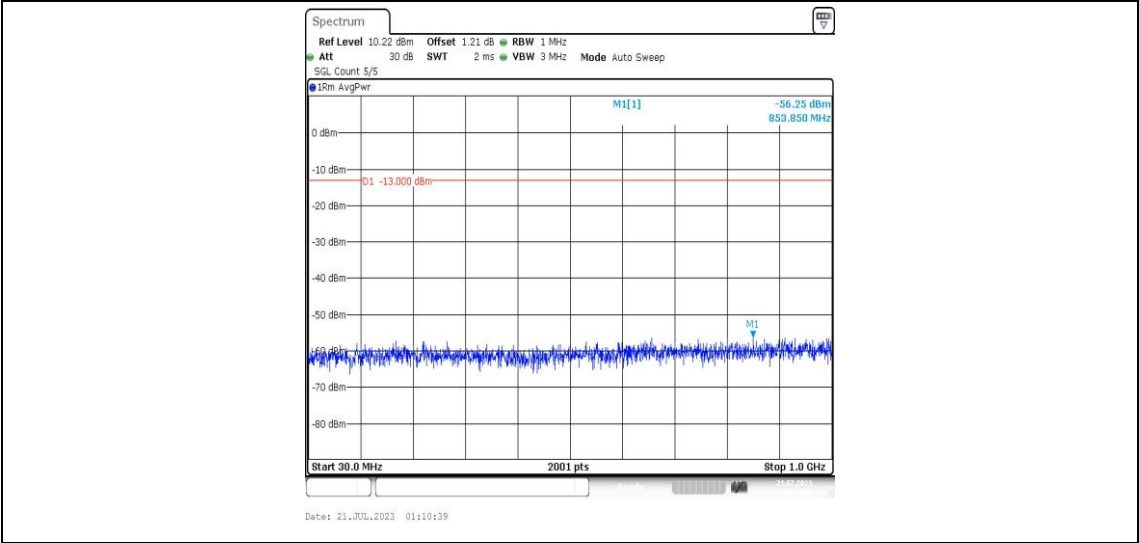
Band25-3MHz-QPSK-26365-1RB#0-Range3:30~1000MHz-PASS
