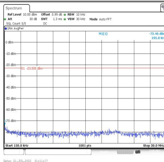
Band25-3MHz-16QAM-26365-1RB#0-Range2:0.15~30MHz-PASS
