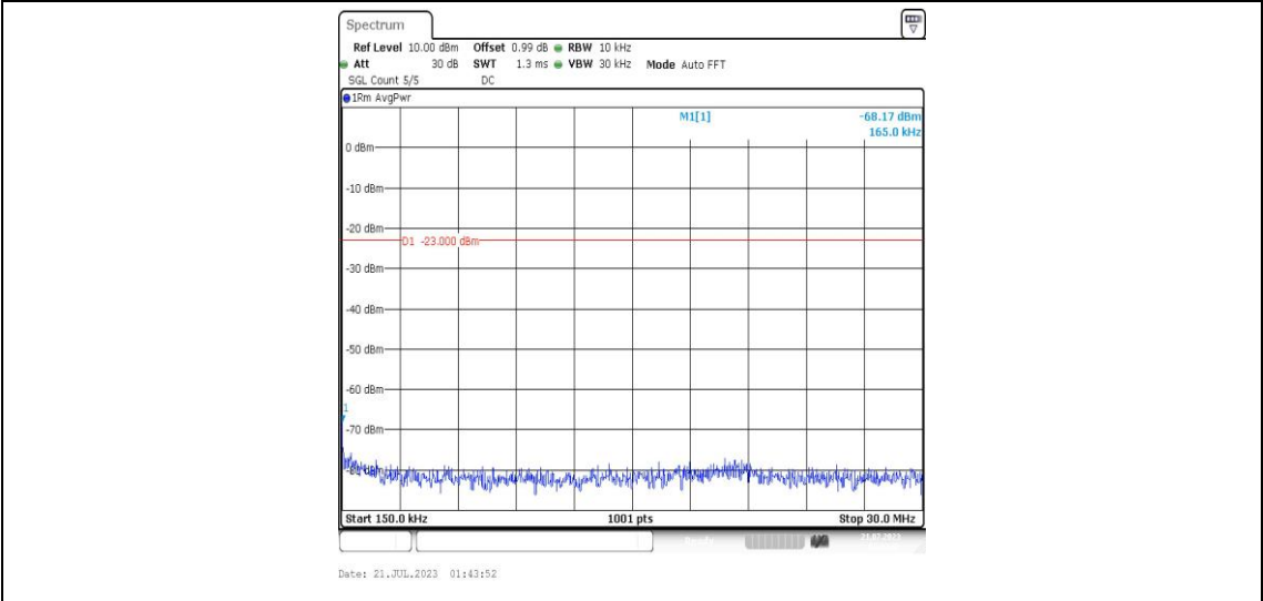
Band25-5MHz-QPSK-26365-1RB#0-Range2:0.15~30MHz-PASS
