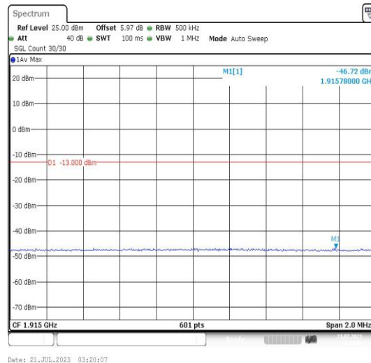
Band25-20MHz-QPSK-26590-1RB#0-PASS
