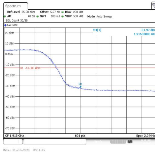
Band25-10MHz-QPSK-26640-50RB#0-PASS
