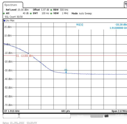
Band25-20MHz-QPSK-26590-100RB#0-PASS
