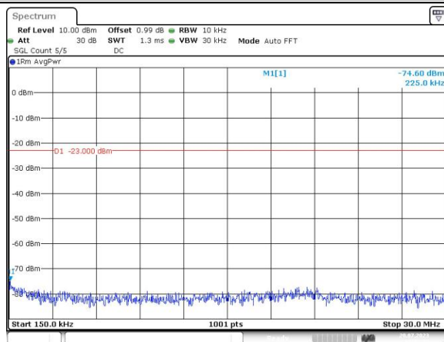
Band12-1.4MHz-QPSK-23017-1RB#0-Range2:0.15~30MHz
