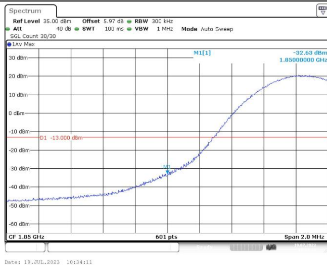
Band2-15MHz-16QAM-18675-1RB#74
