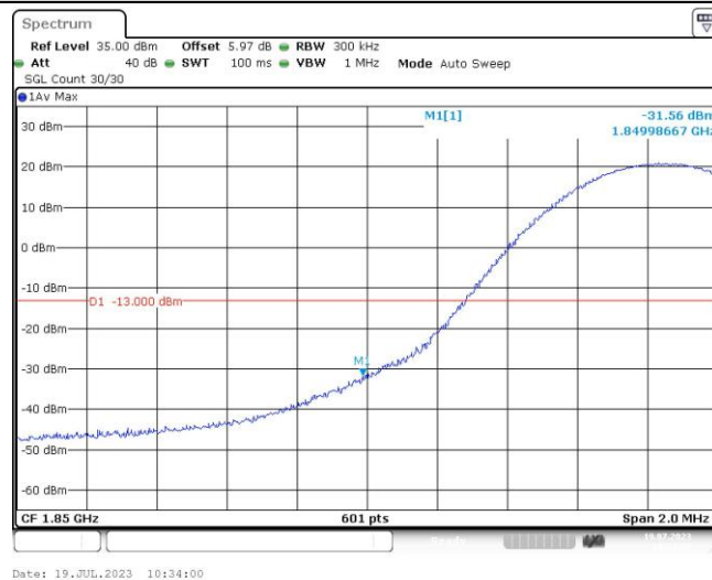
Band2-15MHz-QPSK-18675-1RB#74
