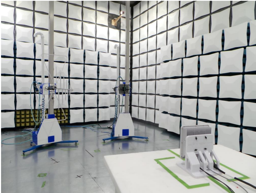
Setup 2. Test Setup <1GHz - SU
