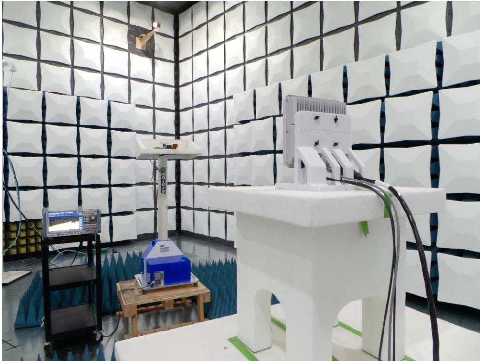
Setup 8. Test Setup >40GHz - SU
