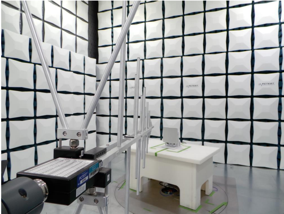
Setup 1. Test Setup <1GHz – SU
