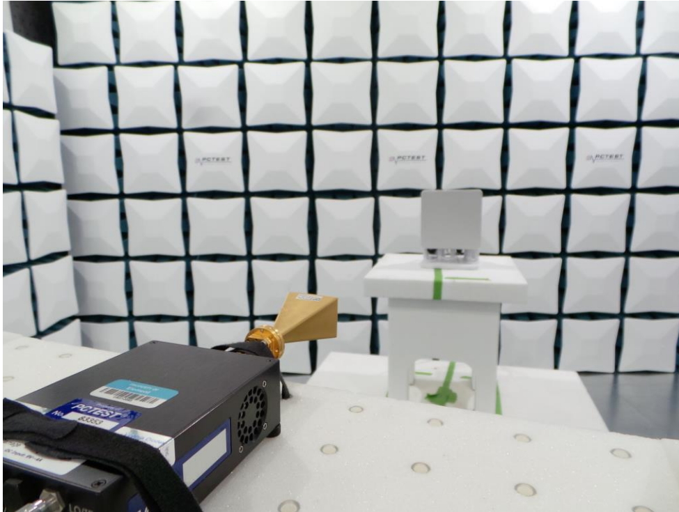
Setup 7. Test Setup >40GHz - SU
