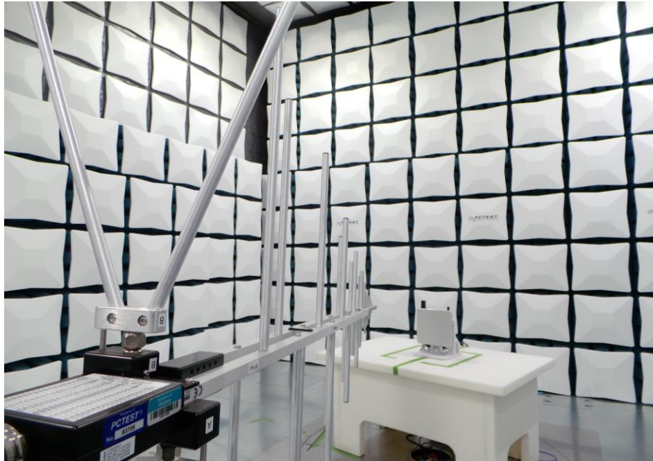
Setup 1. Test Setup <1GHz - DU
