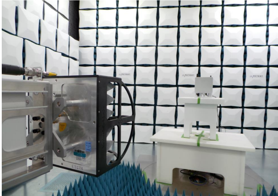
Setup 3. Test Setup 1-18GHz - DU
