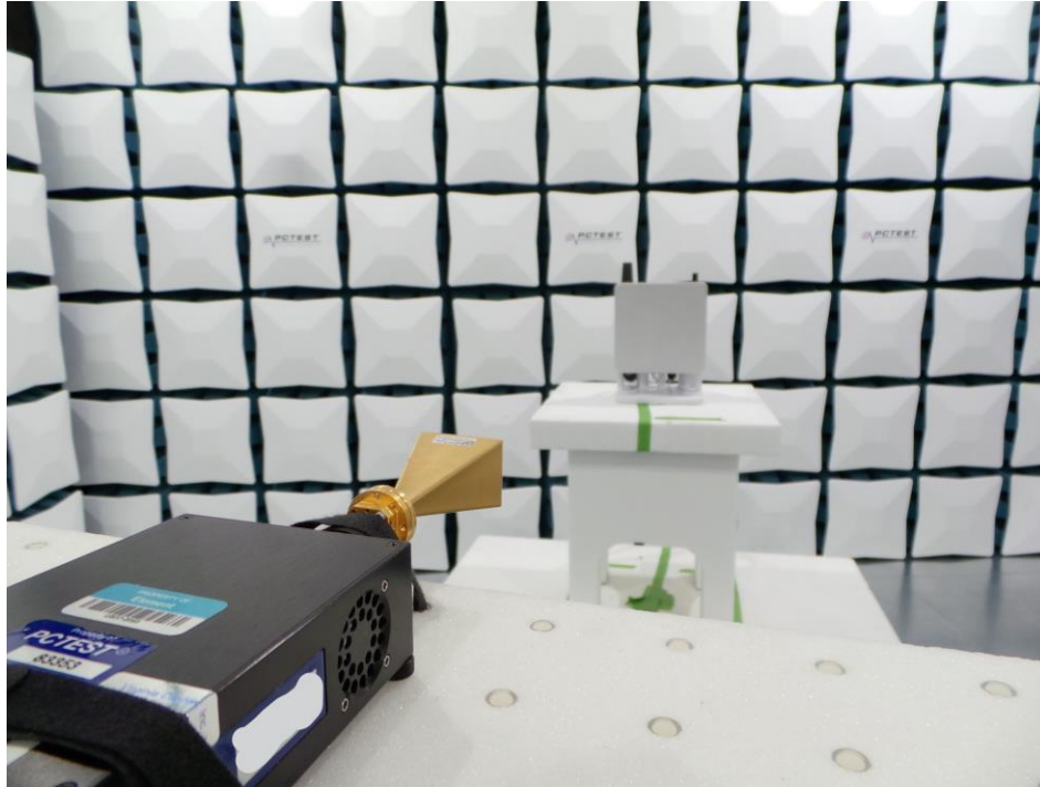
Setup 7. Test Setup >40GHz - DU
