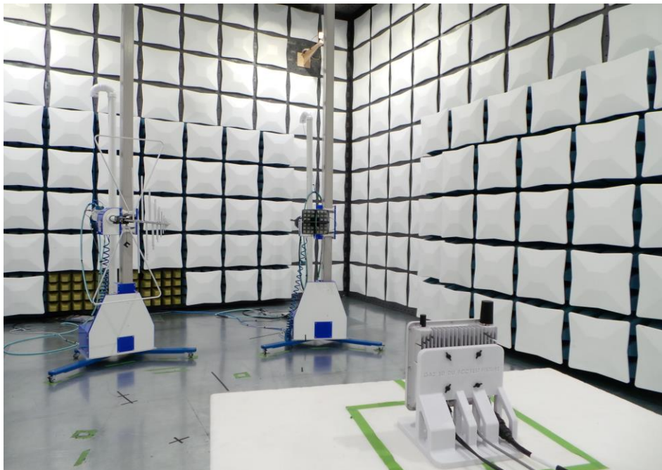
Setup 2. Test Setup <1GHz - DU
