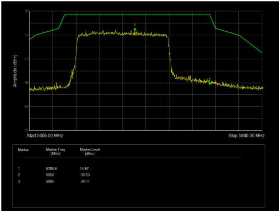
Band Edge NVNT 802.11ax80 5775MHz Low Ant 0
