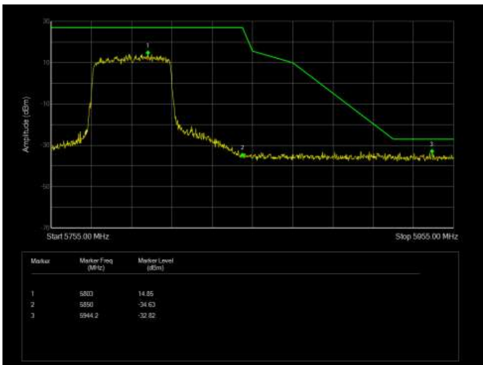
Band Edge NVNT 802.11ax40 5755MHz Low Ant 3
