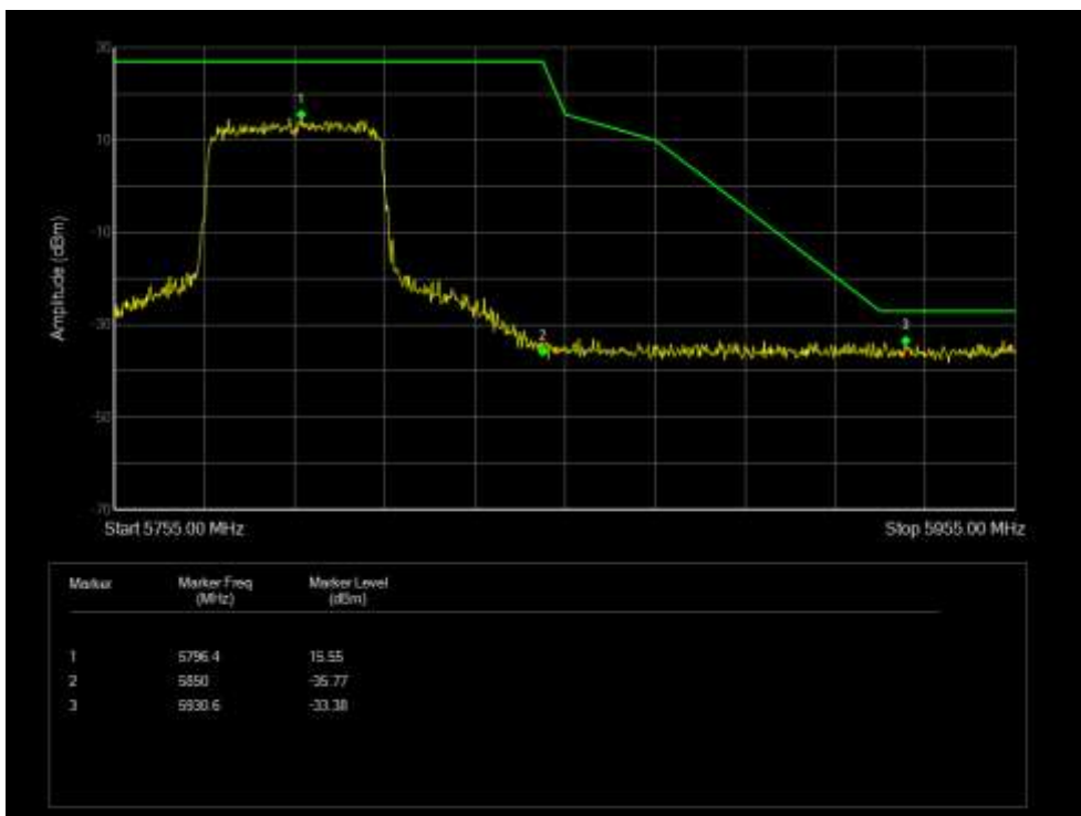
Band Edge NVNT 802.11ax80 5775MHz High Ant 0
