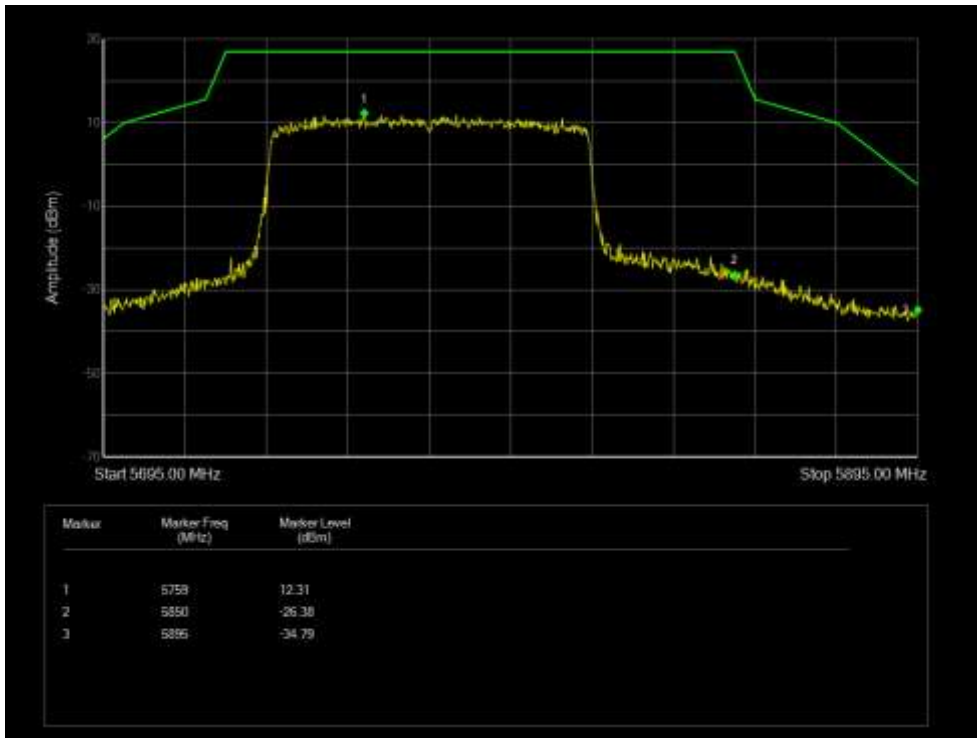
Band Edge NVNT 802.11ax80 5775MHz Low Ant 3
