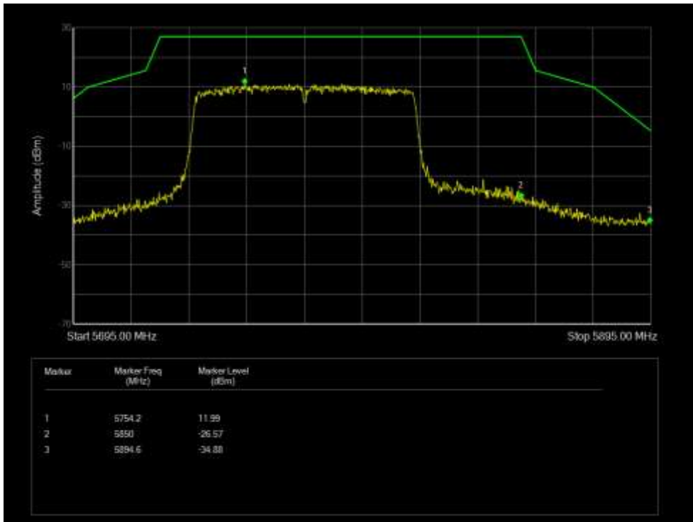
Band Edge NVNT 802.11ac80 5775MHz Low Ant 3
