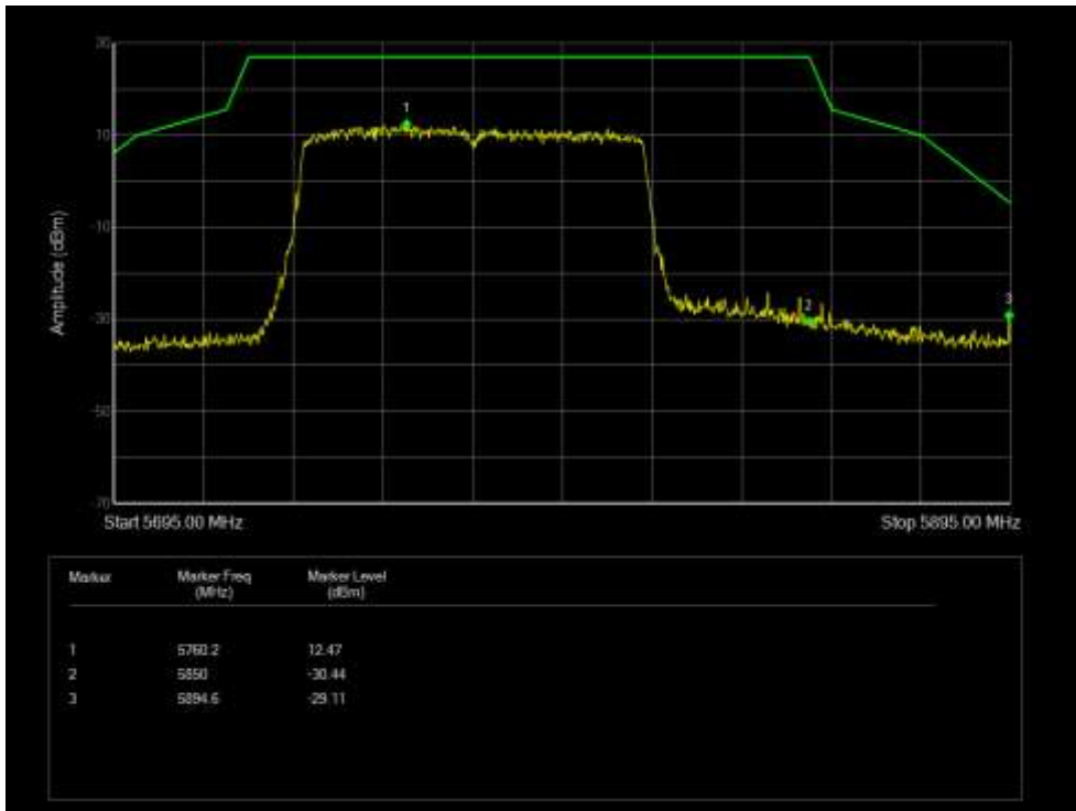
Band Edge NVNT 802.11ac80 5775MHz Low Ant 0
