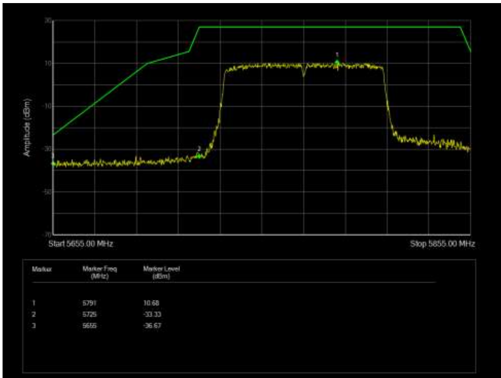
Band Edge NVNT 802.11ac80 5775MHz High Ant 3
