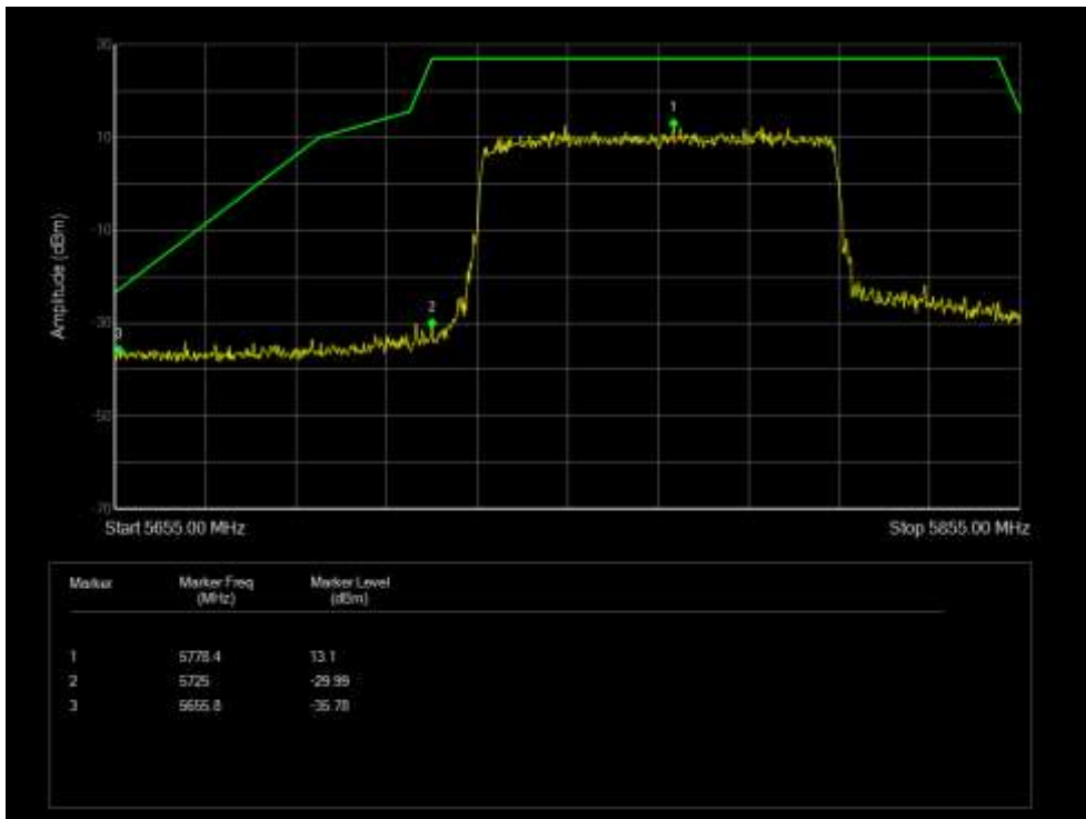
Band Edge NVNT 802.11ax80 5775MHz High Ant 3
