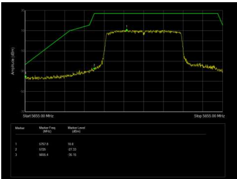
Band Edge NVNT 802.11ax20 5745MHz Low Ant 0
