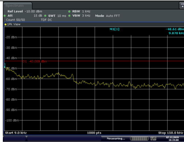
9KHz~150KHz
