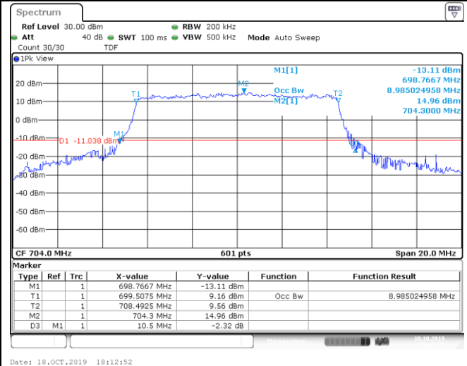
50RB#0
