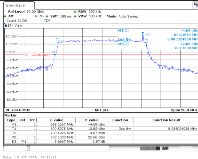
50RB#0
