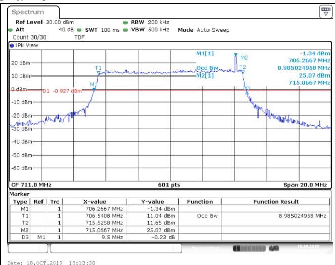
50RB#0
