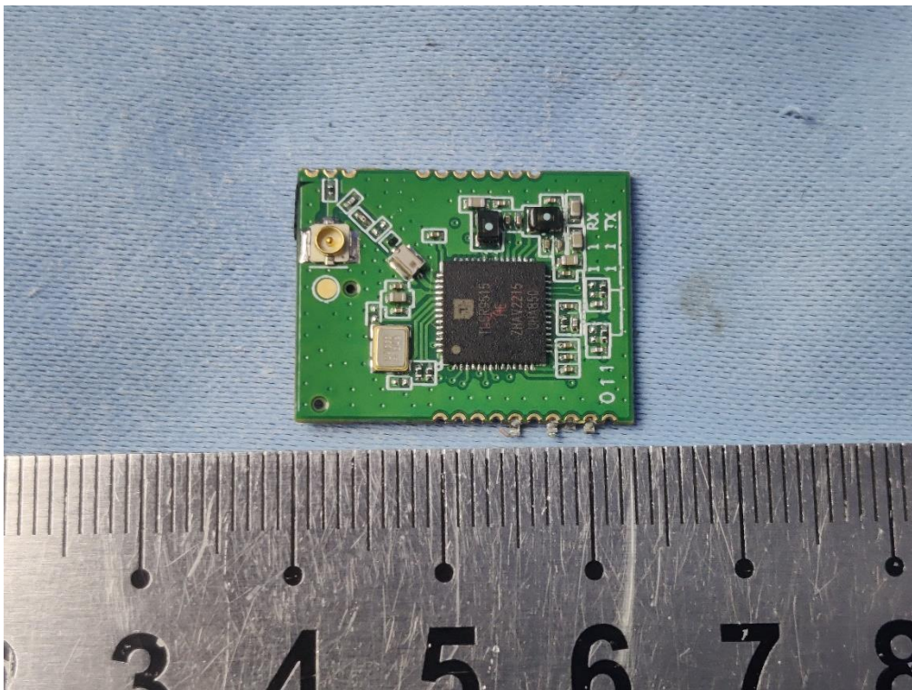
2.4GHz module
