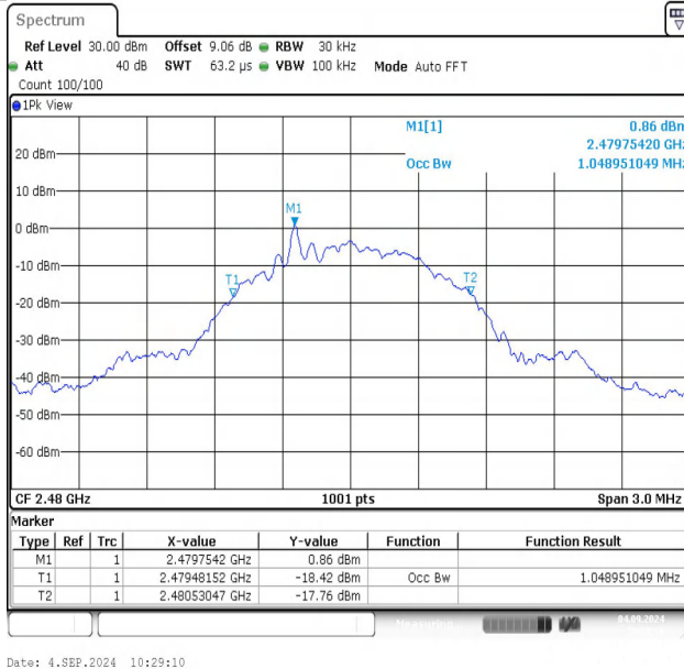
DH5-Ant1-2480
