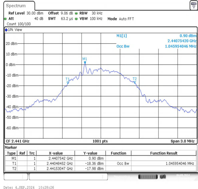
DH5-Ant1-2441
