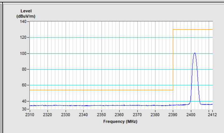
Horizontal (Average)
