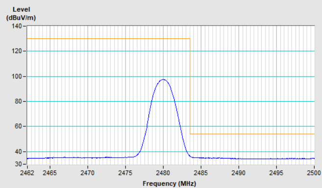
Horizontal (Average)
