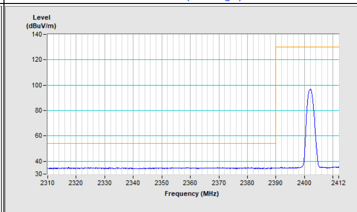
Vertical (Average)
