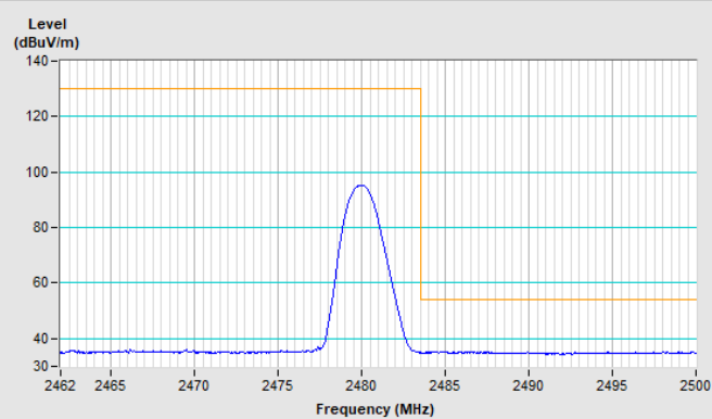
Vertical (Average)
