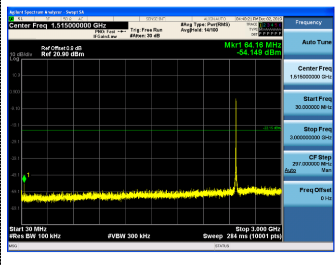
30MHz-3GHz
