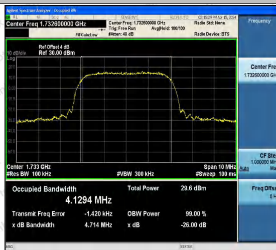
Band4-1413-5-PASS
