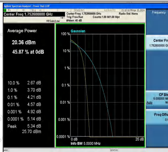
Band4-1513-5-PASS
