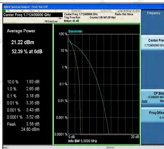
Band4-1312-1-PASS
