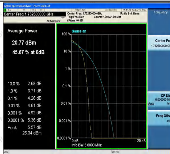
Band4-1413-5-PASS
