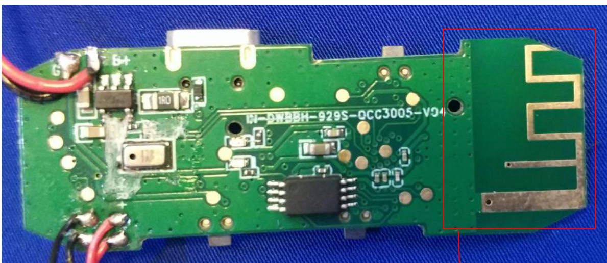
antenna
