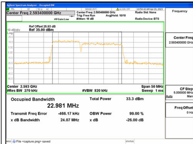
Band41C / 10MHz+15MHz / QPSK/ Mid CH
