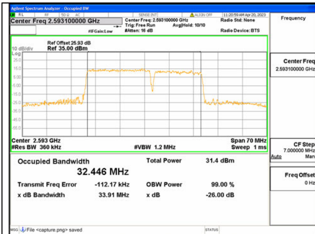
Band41C / 20MHz+15MHz / QPSK/ Mid CH
