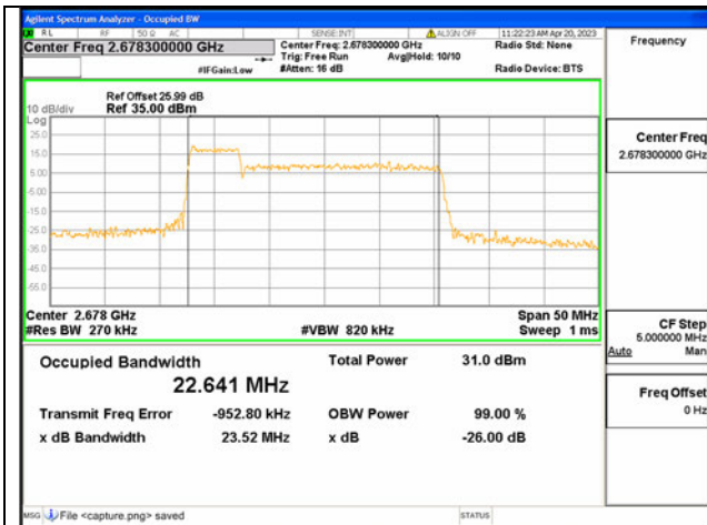
Band41C / 5MHz+20MHz / QPSK/ High CH
