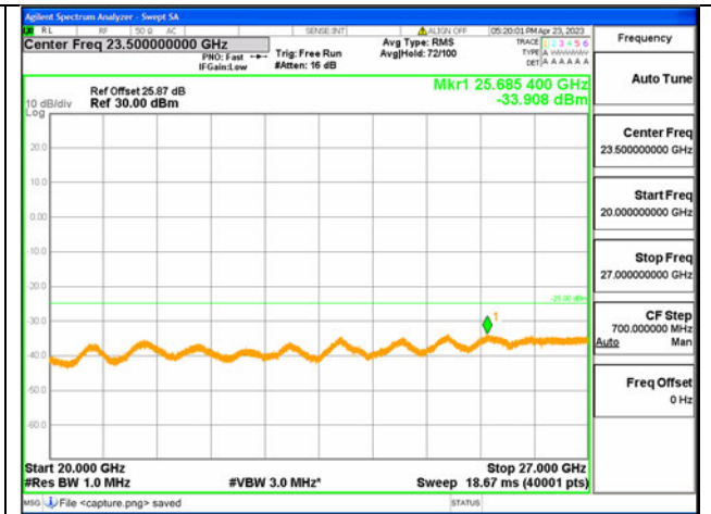
7C-20G-27G / 10+20MHz / QPSK / Low CH / #0-1#99
