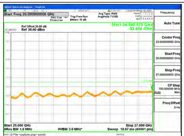
Band41-20G-27G / 15MHz / Low CH / QPSK
