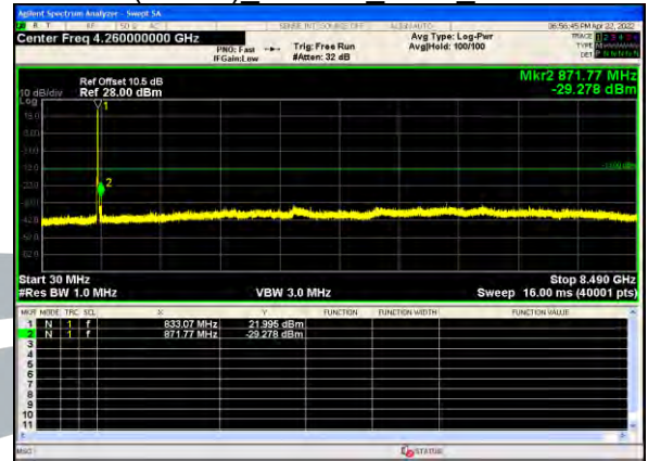
B5(10.0M) QPSK 1RB0 Middle
