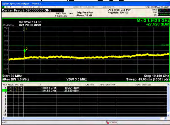
B25(20.0M) 64QAM 1@0 Lowest
