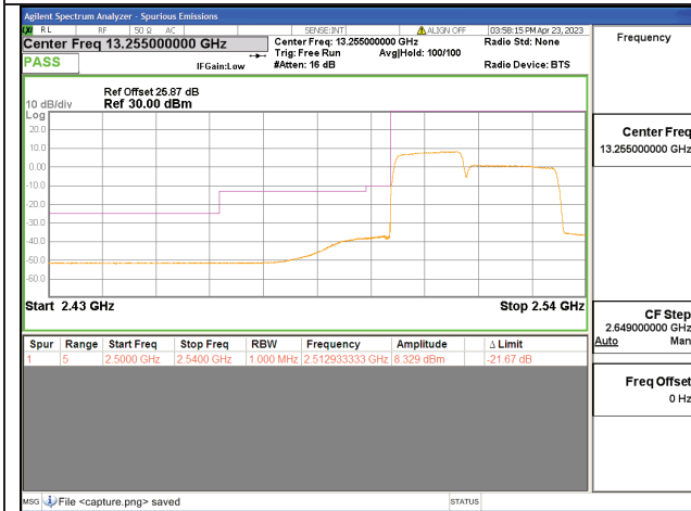
7C / 15+20MHz / Low CH / QPSK / 75#0-100#0
