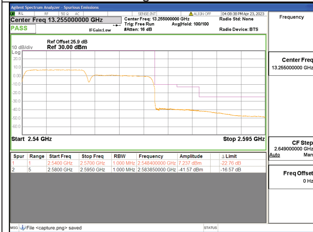
7C / 15+15MHz / High CH / QPSK / 75#0-75#0
