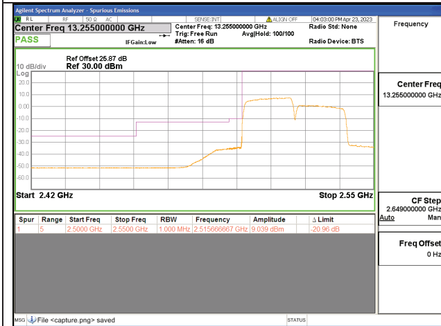
7C / 20+20MHz / Low CH / QPSK / 100#0-100#0
