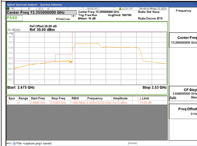
41C / 10+15MHz / Low CH / QPSK / 50#0-75#0
