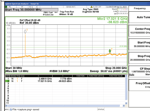
41C-30M-20G / 15+10MHz / QPSK / Low CH / 75#0-50#0
