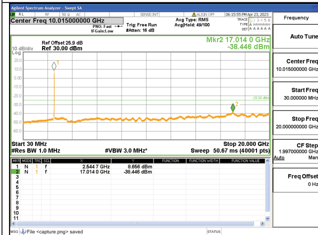
7C-30M-20G / 20+10MHz / QPSK / High CH / 100#0-50#0
