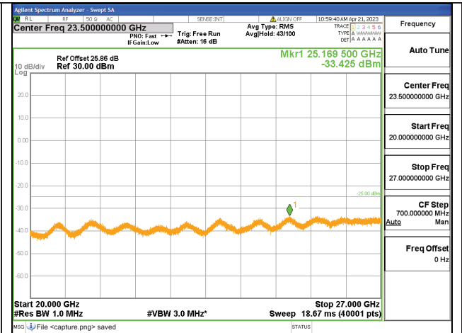
41C-20G-27G / 5+20MHz / QPSK / Low CH / #0-1#99
