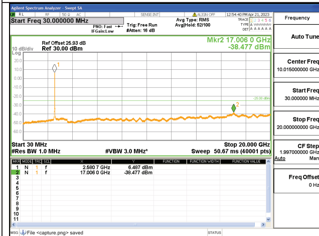
41C-30M-20G / 20+10MHz / QPSK / Mid CH / 100#0-50#0
