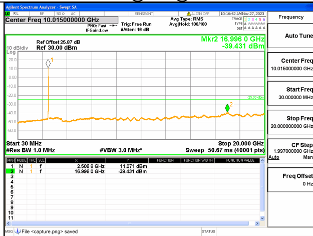
7C-30M-20G / 10+20MHz / QPSK / Low CH / 50@0-100@0
