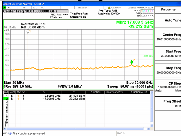
7C-30M-20G / 10+20MHz / QPSK / Low CH / 1@49-1@0
