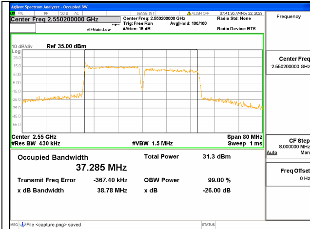
7C / 20+20MHz / QPSK/ High CH
