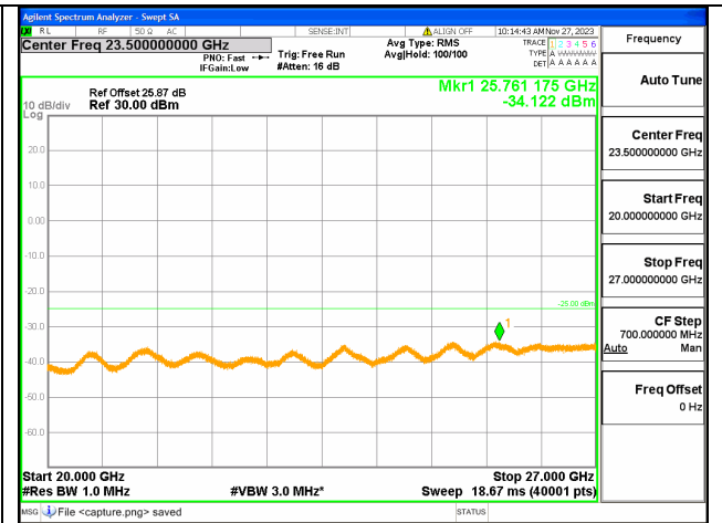
7C-20G-27G / 10+20MHz / QPSK / Low CH / 1@0-1@99
