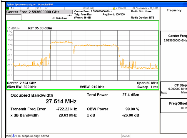
41C / 10+20MHz / QPSK/ Mid CH
