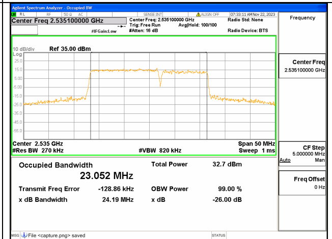
7C / 15+10MHz / 64QAM/ Mid CH
