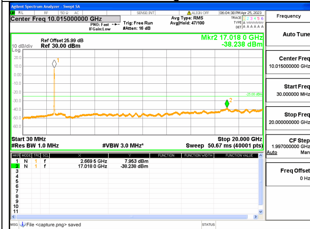
Band41C-30M-20G / 15+15MHz /75RB+75RB/ QPSK / High CH
