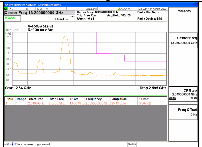
Band7C / 20+10MHz / High CH / QPSK / 1 RB
