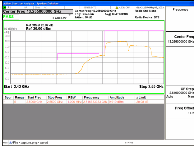
Band7C / 20+20MHz / Low CH / QPSK / 100 RB
