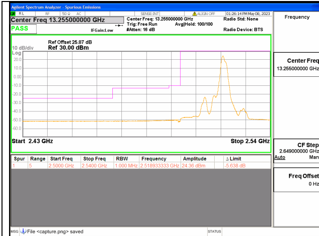
Band7C / 20+10MHz / Low CH / QPSK / 1 RB
