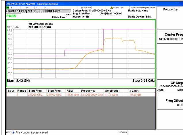
Band7C / 15+10MHz / Low CH / QPSK / 75 RB
