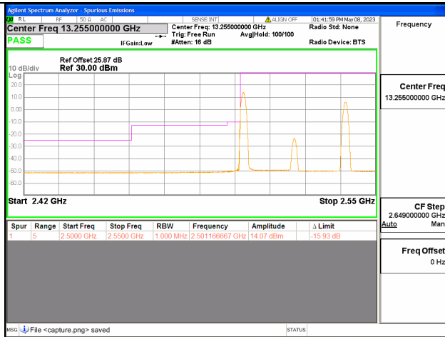
Band7C / 20+20MHz / Low CH / QPSK / 1 RB
