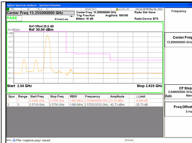
Band7C / 15+10MHz / High CH / QPSK / 1 RB
