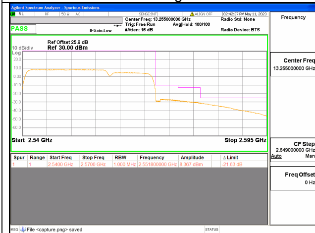
Band7C / 20+10MHz / High CH / QPSK / 100 RB
