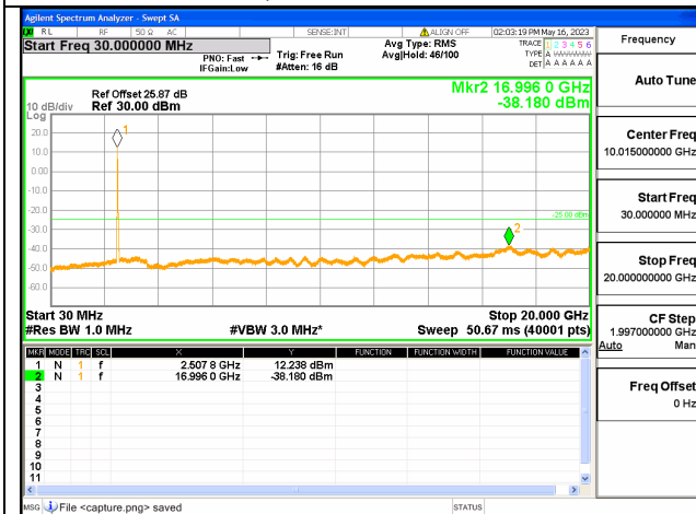
Band7C-30M-20G / 15+15MHz / 75RB+75RB / QPSK / Low CH
