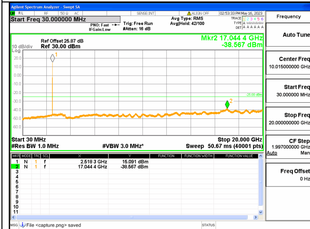
Band7C-30M-20G / 20+20MHz / 1RB+1RB/ QPSK / Low CH
