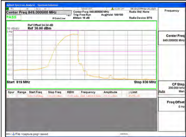
Band26 Part90 / 1.4MHz / High CH / QPSK / 1 RB
