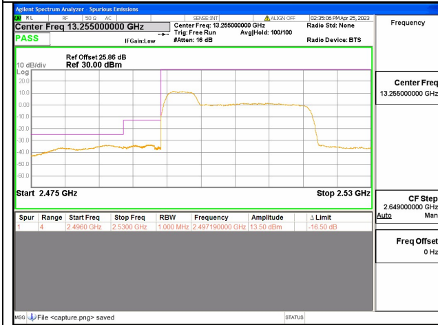
Band41C / 5+20MHz / Low CH / QPSK / 25 RB
