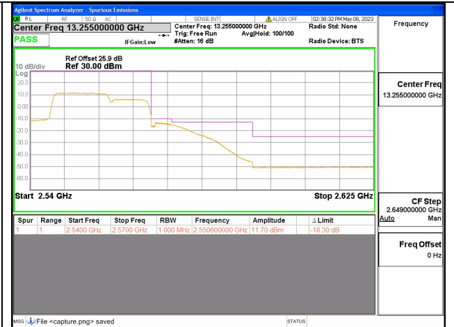
Band7C / 15+10MHz / High CH / QPSK / 75 RB
