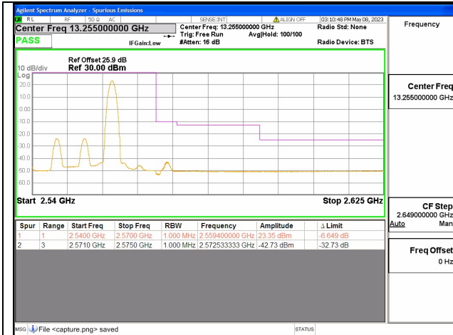
Band7C / 15+10MHz / High CH / QPSK / 1 RB
