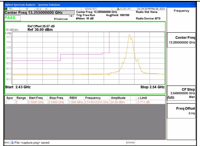
Band7C / 15+20MHz / Low CH / QPSK / 75 RB
