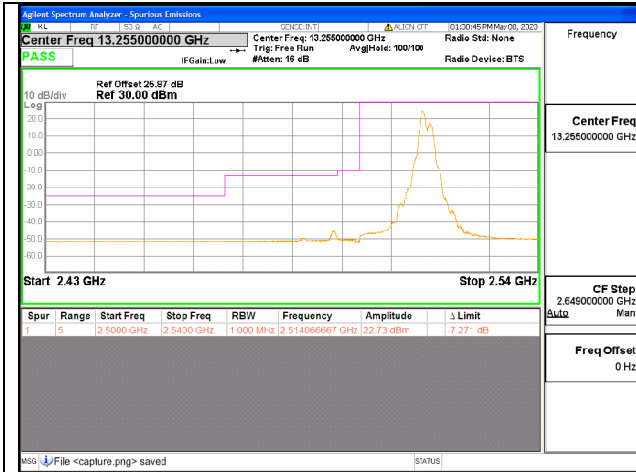
Band7C / 15+15MHz / Low CH / QPSK / 1 RB
