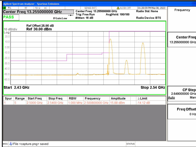
Band7C / 15+10MHz / Low CH / QPSK / 1 RB
