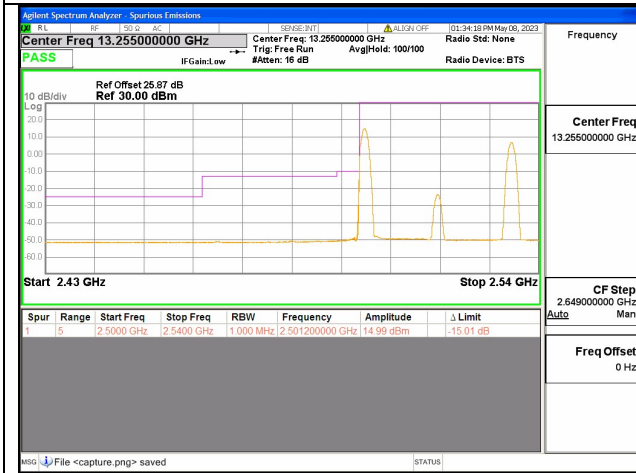
Band7C / 15+20MHz / Low CH / QPSK / 1 RB
