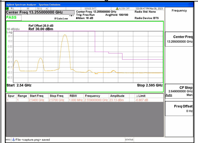
Band7C / 20+10MHz / High CH / QPSK / 50 RB
