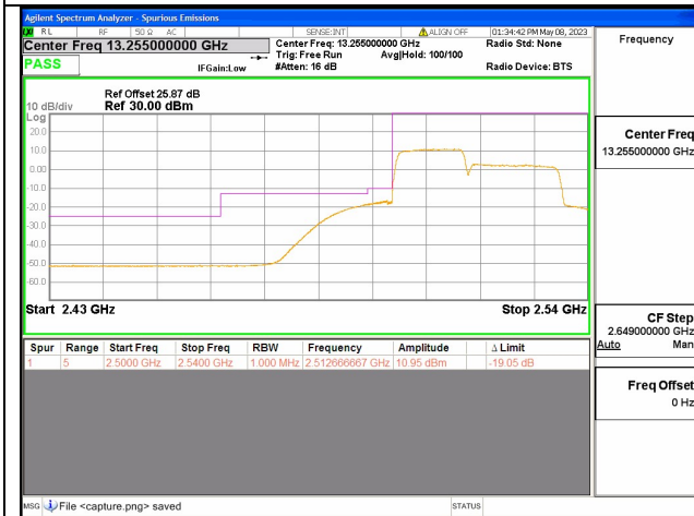
Band7C / 15+20MHz / Low CH / QPSK / 75 RB
