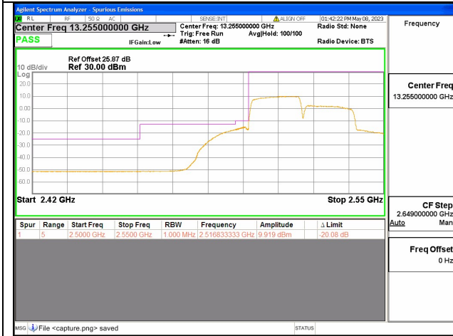
Band7C / 20+20MHz / Low CH / QPSK / 100 RB
