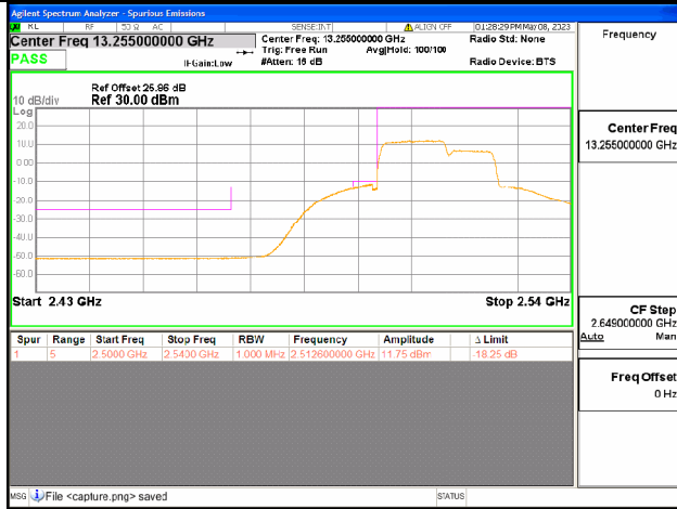
Band7C / 15+10MHz / Low CH / QPSK / 75 RB
