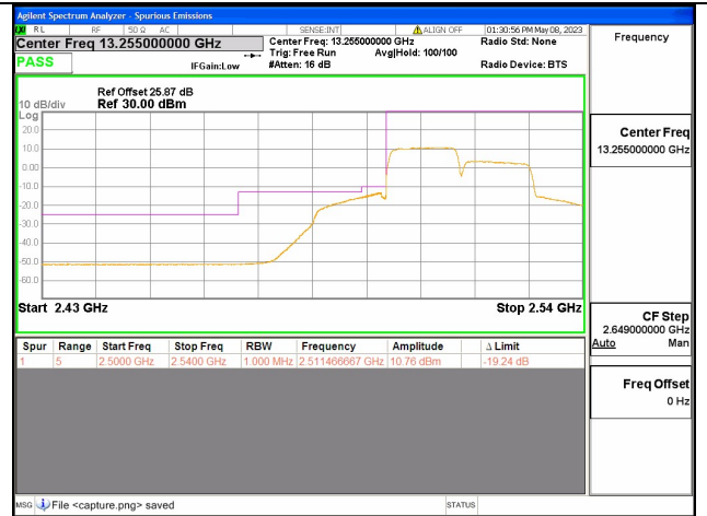
Band7C / 15+15MHz / Low CH / QPSK / 75 RB
