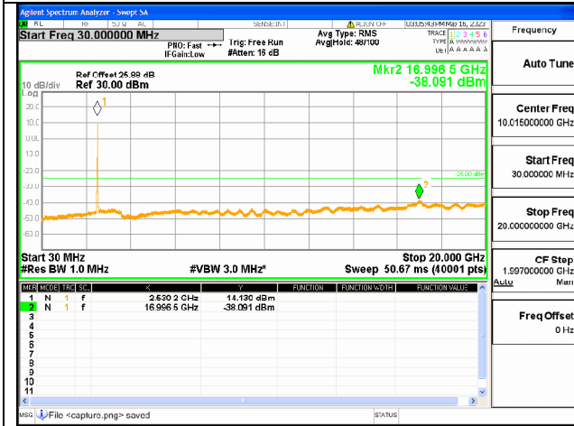
Band7C-30M-20G / 15+10MHz / 75RB+50RB/ QPSK / Mid CH
