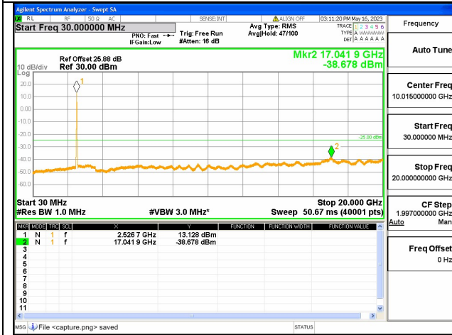
Band7C-30M-20G / 15+15MHz /75RB+75RB/ QPSK / Mid CH
