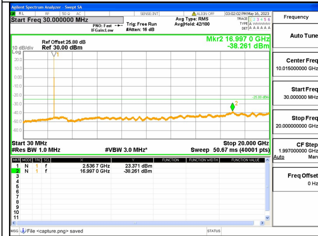
Band7C-30M-20G / 15+10MHz / 1RB+1RB/ QPSK / Mid CH
