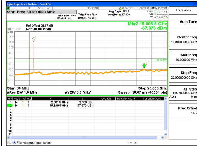
Band7C-30M-20G / 20+15MHz /100RB+75RB/ QPSK / Low CH
