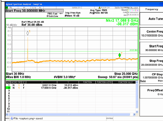
Band7C-30M-20G / 20+10MHz /100RB+50RB/ QPSK / Mid CH
