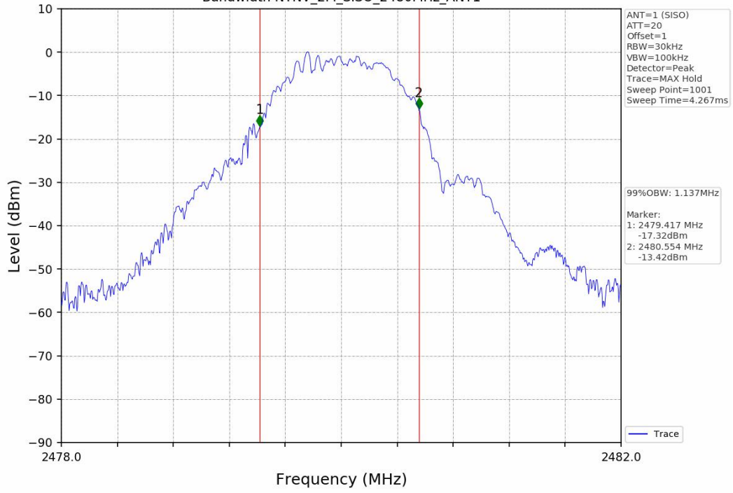
Bandwidth NTVN_2M_SISO_2480MHz_ANT1
